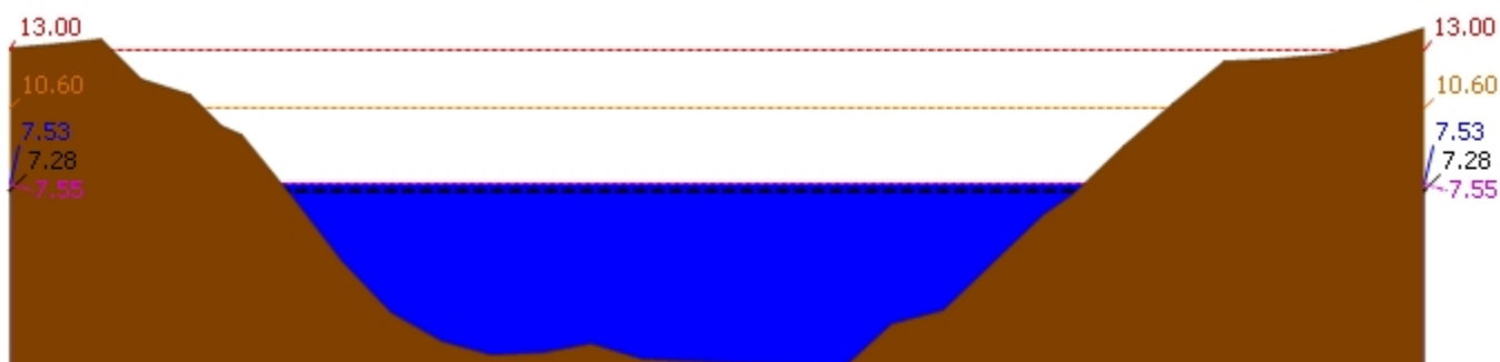
▲ ระดับปัจจุบัน --- ระดับวิกฤติ --- ระดับเฝ้าระวัง ---- เมื่อกาน 7:00 น. - - - - - คาดการณ์ล่วงหน้า 1 วัน สถานี 120106T แม่น้ำป่าสักที่ อ.เสาไห้ ต.ศาลาวิไทย อ.เสาไห้ จ.สระบุรี ระดับน้ำ 7.53 ม.รทก.
