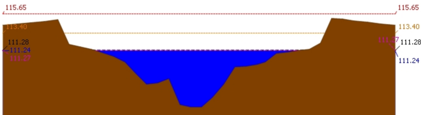
▲ ระดับปัจจุบัน --- ระดับวิกฤติ --- ระดับเฝ้าระวัง ---- เมื่อกาน 7:00 น. - - - - - คาดการณ์ล่วงหน้า 1 วัน สถานี 120107T แม่น้ำป่าสักที่ อ.เมืองเพชรบูรณ์ ต.นาป่า อ.เมือง จ.เพชรบูรณ์ ระดับน้ำ 111.24 ม.รทก.
