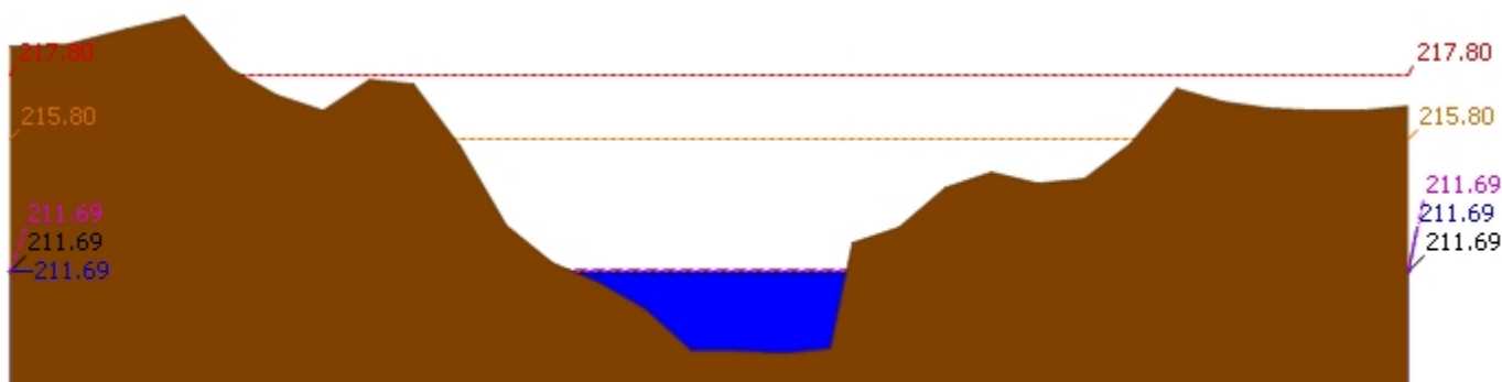
▲ ระดับปัจจุบัน --- ระดับวิกฤติ --- ระดับเฝ้าระวัง ---- เมื่อกาน 7:00 น. - - - - - คาดการณ์ล่วงหน้า 1 วัน สถานี 120205T แม่น้ำป่าสักที่บ้านอุมกะทาด ต.ศิลา อ.หล่มเก่า จ.เพชรบูรณ์ ระดับน้ำ 211.69 ม.รทก.
