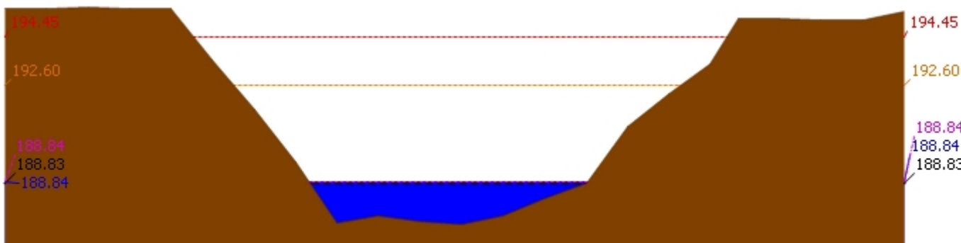
▲ ระดับปัจจุบัน --- ระดับวิกฤติ --- ระดับเฝ้าระวัง ---- เมื่อกาน 7:00 น. - - - - - คาดการณ์ล่วงหน้า 1 วัน สถานี 120901T ห้วยมวกเหล็กที่ อ.มวกเหล็ก ต.มวกเหล็ก อ.มวกเหล็ก จ.สระบุรี ระดับน้ำ 188.84 ม.รทก.
