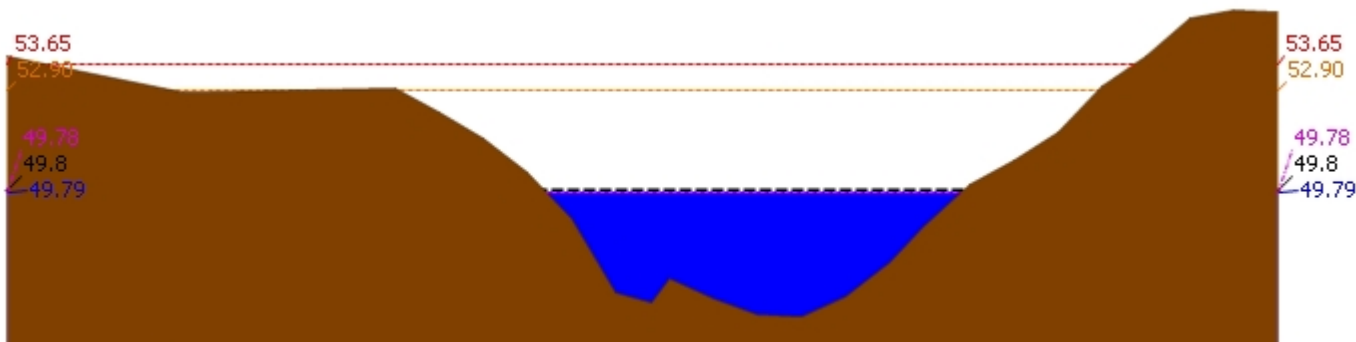
▲ ระดับปัจจุบัน --- ระดับวิกฤติ --- ระดับเฝ้าระวัง ---- เมื่อกาน 7:00 น. - - - - - คาดการณ์ล่วงหน้า 1 วัน สถานี 120113T แม่น้ำป่าสักที่บ้านเขาค้าง ต.คลองกระจิง อ.ศรีเทพ จ.เพชรบูรณ์ ระดับน้ำ 49.79 ม.รทก.
