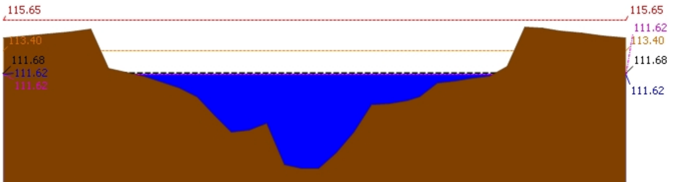
▲ ระดับปัจจุบัน --- ระดับวิกฤติ --- ระดับฝายระวัง - - - - - เมื่อวาน 7:00 น. - - - - - คาดการณ์ล่วงหน้า 1 วัน สถานี 120107T แม่น้ำป่าสักที่ อ.เมืองเพชรบูรณ์ ต.นาป่า อ.เมือง จ.เพชรบูรณ์ ระดับน้ำ 111.62 ม.รทก.
