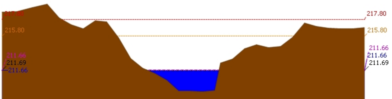
▲ ระดับปัจจุบัน --- ระดับวิกฤติ --- ระดับฝายระวัง - - - - - เมื่อวาน 7:00 น. - - - - - คาดการณ์ล่วงหน้า 1 วัน สถานี 120205T แม่น้ำป่าสักที่บ้านอุมกะทาด ต.ศิลา อ.หล่มเก่า จ.เพชรบูรณ์ ระดับน้ำ 211.66 ม.รทก.
