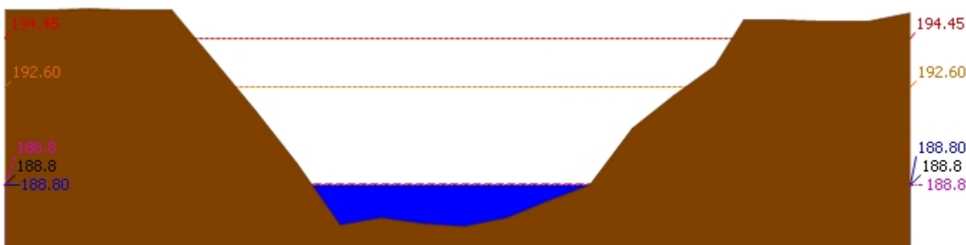
▲ ระดับปัจจุบัน --- ระดับวิกฤติ --- ระดับฝายระวัง ---- เมื่อวาน 7:00 น. - - - - คาดการณ์ล่วงหน้า 1 วัน สถานี 120901T ห้วยมวกเหล็กที่ อ.มวกเหล็ก ต.มวกเหล็ก อ.มวกเหล็ก จ.สระบุรี ระดับน้ำ 188.80 ม.รทก.
