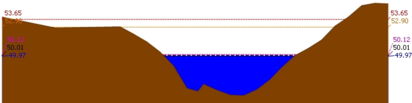
▲ ระดับปัจจุบัน --- ระดับวิกฤติ --- ระดับฝายระวัง ---- เมื่อวาน 7:00 น. - - - - คาดการณ์ล่วงหน้า 1 วัน สถานี 120113T แม่น้ำป่าสักที่บ้านเขาค้าง ต.คลองกระจิง อ.ศรีเทพ จ.เพชรบูรณ์ ระดับน้ำ 49.97 ม.รทก.
