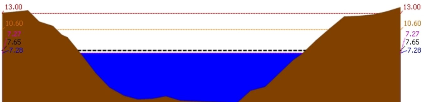
▲ ระดับปัจจุบัน --- ระดับวิกฤติ --- ระดับฝายระวัง ---- เมื่อกาน 7:00 น. - - - - คาดการณ์ล่วงหน้า 1 วัน สถานี 120106T แม่น้ำป่าสักที่ อ.เสนาไห้ ต.ศาลาวิไทย อ.เสนาไห้ จ.สระบุรี ระดับน้ำ 7.28 ม.รทก.
