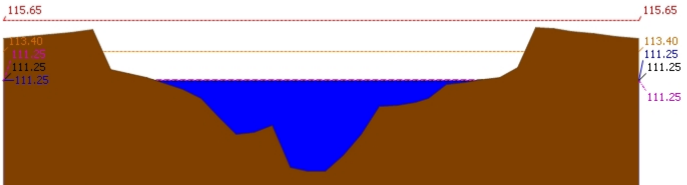
▲ ระดับปัจจุบัน --- ระดับวิกฤติ --- ระดับฝายระวัง ---- เมื่อกาน 7:00 น. - - - - คาดการณ์ล่วงหน้า 1 วัน สถานี 120107T แม่น้ำป่าสักที่ อ.เมืองเพชรบูรณ์ ต.นาป่า อ.เมือง จ.เพชรบูรณ์ ระดับน้ำ 111.25 ม.รทก.
