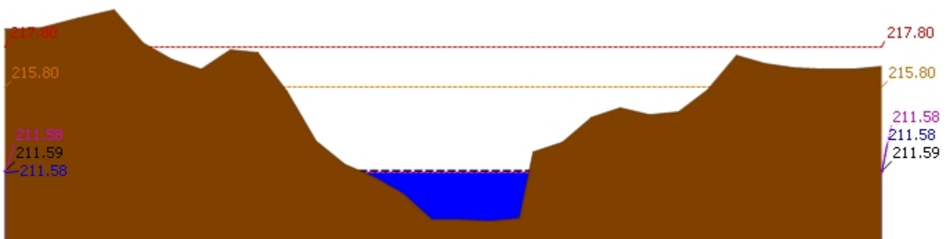
▲ ระดับปัจจุบัน --- ระดับวิกฤติ --- ระดับฝายระวัง ---- เมื่อกาน 7:00 น. - - - - คาดการณ์ล่วงหน้า 1 วัน สถานี 120205T แม่น้ำป่าสักที่บ้านอุมกะทาด ต.ศิลา อ.หล่มเก่า จ.เพชรบูรณ์ ระดับน้ำ 211.58 ม.รทก.
