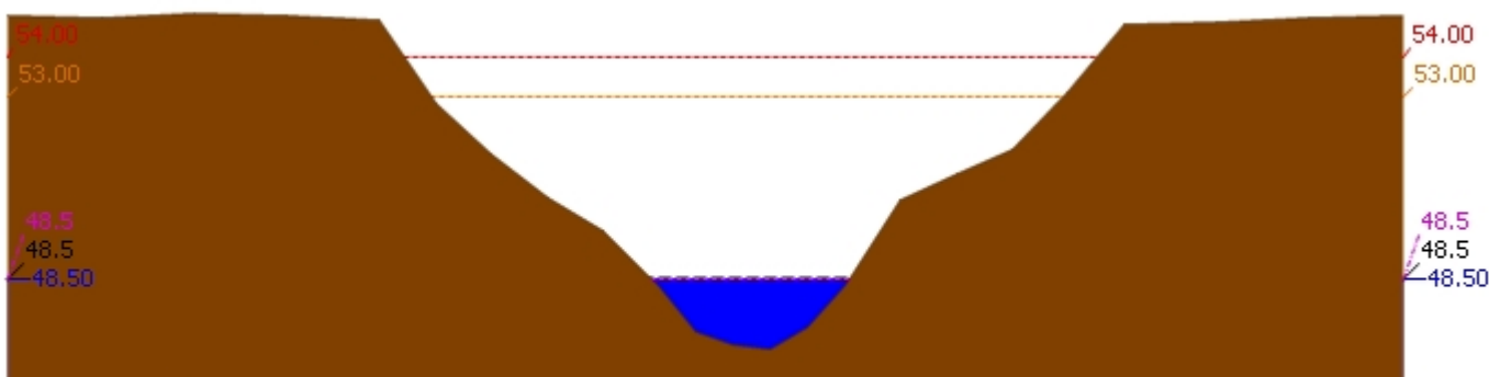
▲ ระดับปัจจุบัน --- ระดับวิกฤติ --- ระดับเฝ้าระวัง ---- เมื่อกาน 7:00 น. - - - - คาดการณ์ล่วงหน้า 1 วัน สถานี 120702T ลำสนธิที่บ้านท่าช้าง ต.หนองขาหย่าง อ.ชัยบาดาล จ.ลพบุรี ระดับน้ำ 48.50 ม.รทก.
