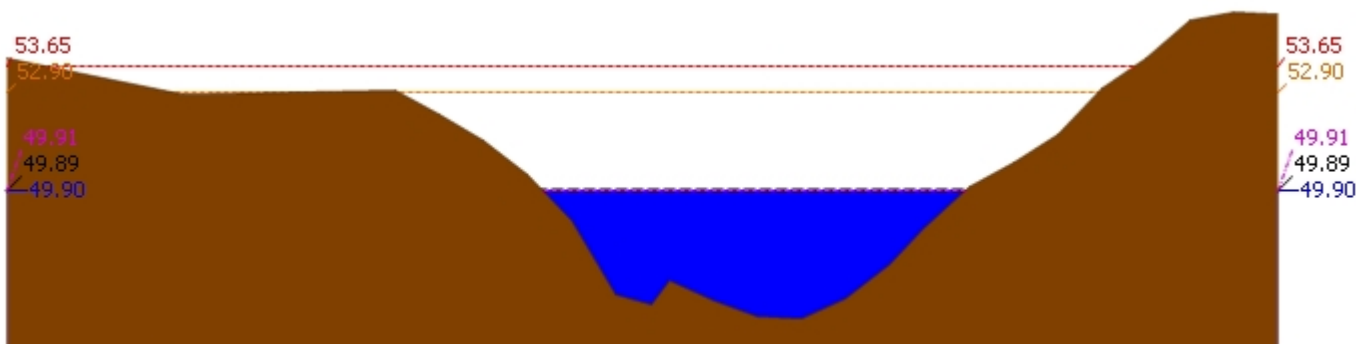
▲ ระดับปัจจุบัน --- ระดับวิกฤติ --- ระดับเฝ้าระวัง ---- เมื่อกาน 7:00 น. - - - - คาดการณ์ล่วงหน้า 1 วัน สถานี 120113T แม่น้ำป่าสักที่บ้านเขาค้าง ต.คลองกระจิง อ.ศรีเทพ จ.เพชรบูรณ์ ระดับน้ำ 49.90 ม.รทก.
