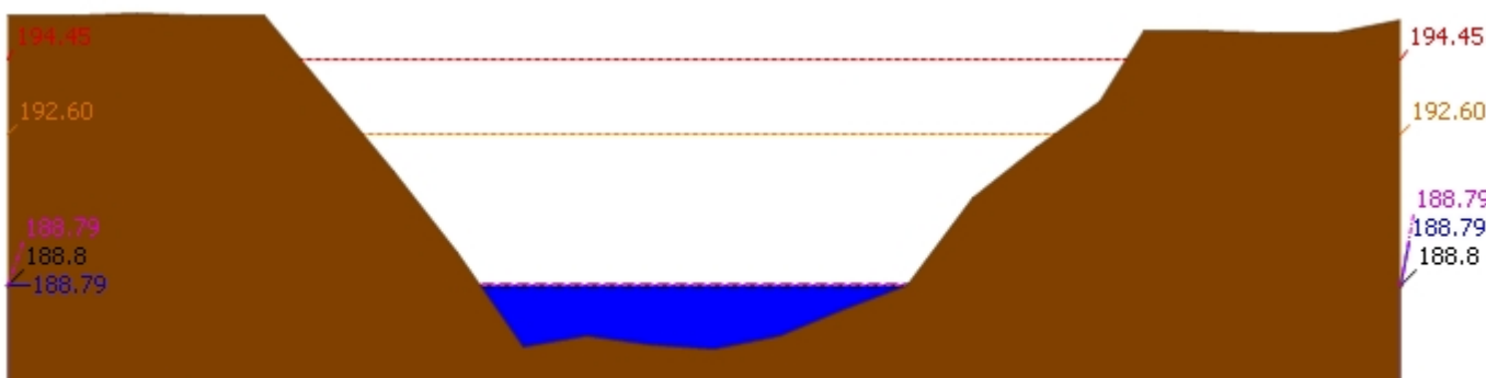
▲ ระดับปัจจุบัน --- ระดับวิกฤติ --- ระดับเฝ้าระวัง ---- เมื่อกาน 7:00 น. - - - - คาดการณ์ล่วงหน้า 1 วัน สถานี 120901T ห้วยมวกเหล็กที่ อ.มวกเหล็ก ต.มวกเหล็ก อ.มวกเหล็ก จ.สระบุรี ระดับน้ำ 188.79 ม.รทก.
