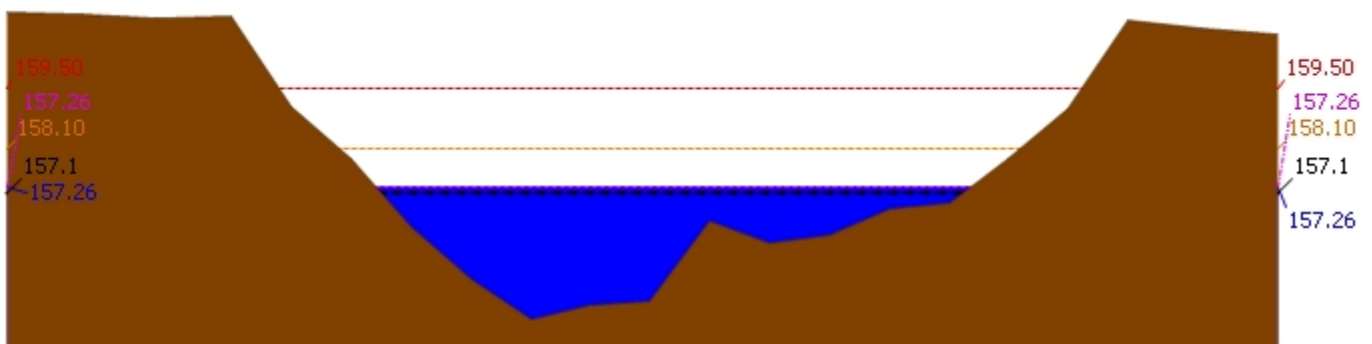
▲ ระดับปัจจุบัน ----- ระดับวิกฤติ ----- ระดับฝายระวัง ----- เมื่อวาน 7:00 น. ----- คาดการณ์ล่วงหน้า 1 วัน สถานี 120305T หัวน้ำพุอยู่ที่ อ.หล่มเก่า ต.หล่มเก่า อ.หล่มเก่า จ.เพชรบูรณ์ ระดับน้ำ 157.26 ม.รทก.
