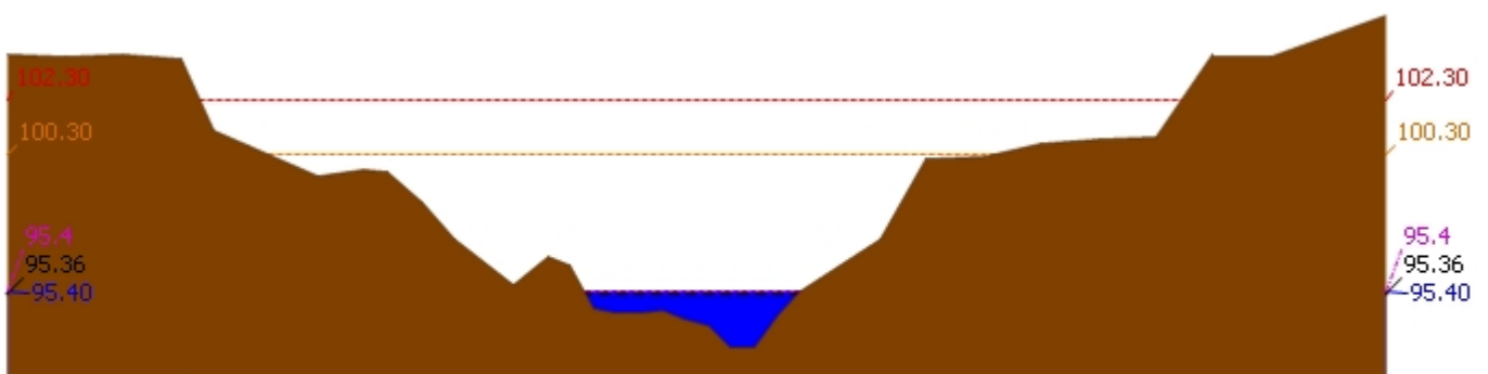
▲ ระดับปัจจุบัน ----- ระดับวิกฤติ ----- ระดับฝายระวัง ----- เมื่อวาน 7:00 น. ----- คาดการณ์ล่วงหน้า 1 วัน สถานี 120112T แม่น้ำป่าสักที่บ้านหนองแหวน ต.วังมะข่อ อ.เมือง จ.เพชรบูรณ์ ระดับน้ำ 95.40 ม.รทก.
