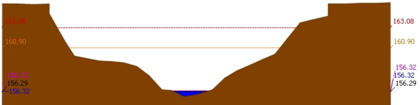
▲ ระดับปัจจุบัน ----- ระดับวิกฤติ ----- ระดับฝายระวัง ----- เมื่อวาน 7:00 น. ----- คาดการณ์ล่วงหน้า 1 วัน สถานี 120105T แม่น้ำป่าสักที่บ้านวังมเหนื่อ ต.ท่าอินดู อ.หล่มสัก จ.เพชรบูรณ์ ระดับน้ำ 156.32 ม.รทก.
