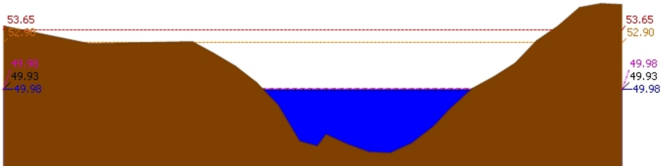
▲ ระดับปัจจุบัน --- ระดับวิกฤติ --- ระดับเฝ้าระวัง ---- เมื่อวาน 7:00 น. - - - - - คาดการณ์ล่วงหน้า 1 วัน สถานี 120113T แม่น้ำป่าสักที่บ้านเขาค้าง ต.คลองกระจิง อ.ศรีเทพ จ.เพชรบูรณ์ ระดับน้ำ 49.98 ม.รทก.
