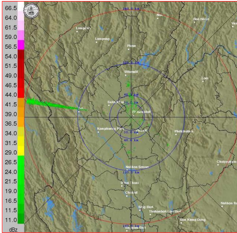
ภาพเรดาร์ตรวจอากาศ “พิชญ์โลก” ณ วันที่ 20 พฤศจิกายน 2561 (ที่มา : กรมอุตุนิยมวิทยา)
