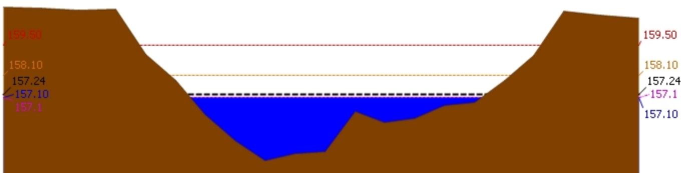
▲ ระดับปัจจุบัน ---- ระดับวิกฤติ - - - - ระดับเฟิาระวัง ---- เมือวาน 7:00 น. - - - - คาดการล้่วงหน้า 1 วัน สถานี 120305T หัวน้ำพุท้ อ.หล่มเก่า ต.หล่มเก่า อ.หล่มเก่า จ.เพชรบูรณ์ ระดับน้ำ 157.10 ม.รทก.
