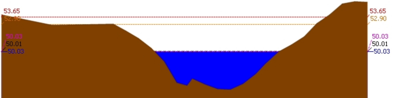
▲ ระดับปัจจุบัน --- ระดับวิกฤติ --- ระดับเฝ้าระวัง ---- เมื่อวาน 7:00 น. - - - - - คาดการณ์ล่วงหน้า 1 วัน สถานี 120113T แม่น้ำป่าสักที่บ้านเขาค้าง ต.คลองกระจิง อ.ศรีเทพ จ.เพชรบูรณ์ ระดับน้ำ 50.03 ม.รทก.
