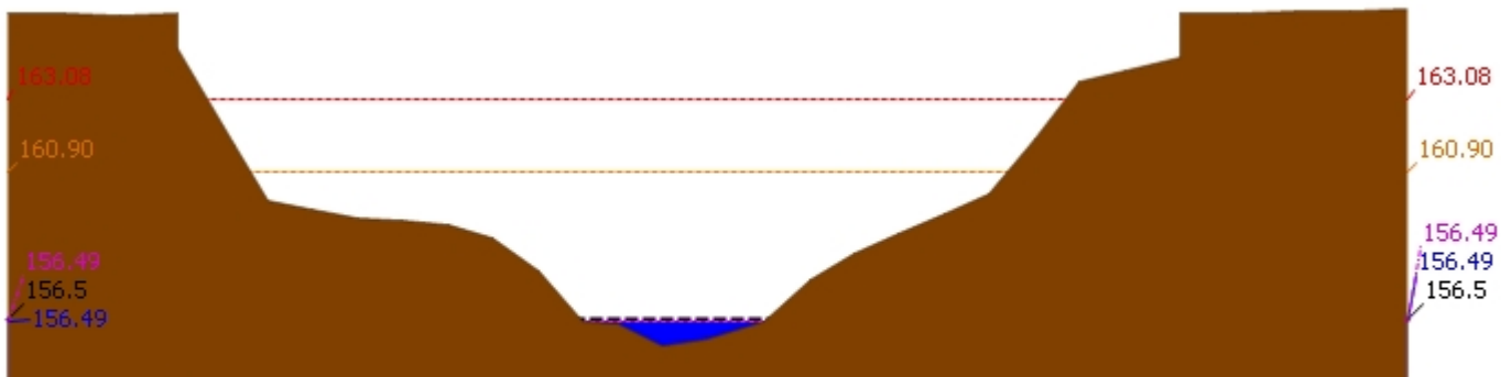
▲ ระดับปัจจุบัน ---- ระดับวิกฤติ - - - - ระดับเฟิาระวัง ---- เมือวาน 7:00 น. - - - - คาดการล้่วงหน้า 1 วัน สถานี 120105T แม่น้ำป่าสักที่บ้านวังมเหนือ ต.ท่าอิบลู อ.หล่มสัก จ.เพชรบูรณ์ ระดับน้ำ 156.49 ม.รทก.
