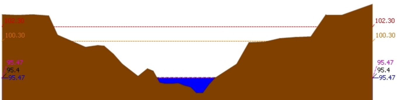
▲ ระดับปัจจุบัน ---- ระดับวิกฤติ - - - - ระดับเฟิาระวัง ---- เมือวาน 7:00 น. - - - - คาดการล้่วงหน้า 1 วัน สถานี 120112T แม่น้ำป่าสักที่บ้านหนองแหวน ต.วังมะช่อ อ.เมือง จ.เพชรบูรณ์ ระดับน้ำ 95.47 ม.รทก.
