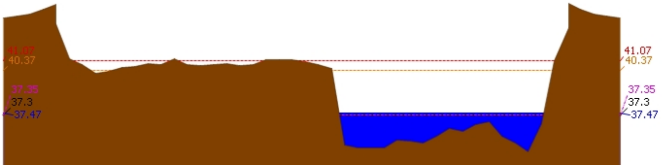
▲ ระดับปัจจุบัน --- ระดับวิกฤติ --- ระดับเฝ้าระวัง ---- เมื่อกวาน 7:00 น. - - - - คาดการณ์ล่วงหน้า 1 วัน สถานี 060110T แม่น้ำปิงที่บ้านบางแก้ว ต.บางแก้ว อ.บรรพตพิสัย จ.นครสวรรค์ ระดับน้ำ 37.47 ม.รทก.
