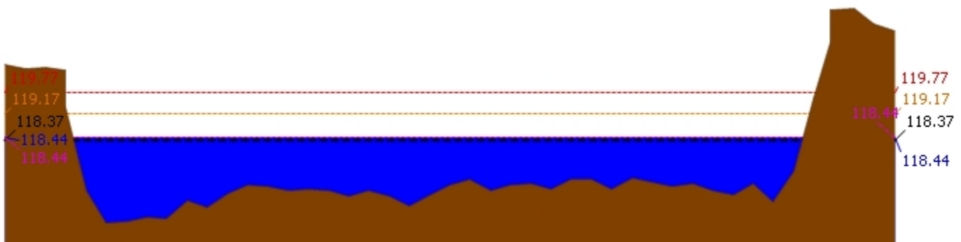
▲ ระดับปัจจุบัน --- ระดับวิกฤติ --- ระดับเฝ้าระวัง ---- เมื่อกวาน 7:00 น. - - - - คาดการณ์ล่วงหน้า 1 วัน สถานี 060111T แม่น้ำปิงที่บ้านปากร่องห้วยจี่ ต.ตากออก อ.บ้านตาก จ.ตาก ระดับน้ำ 118.44 ม.รทก.
