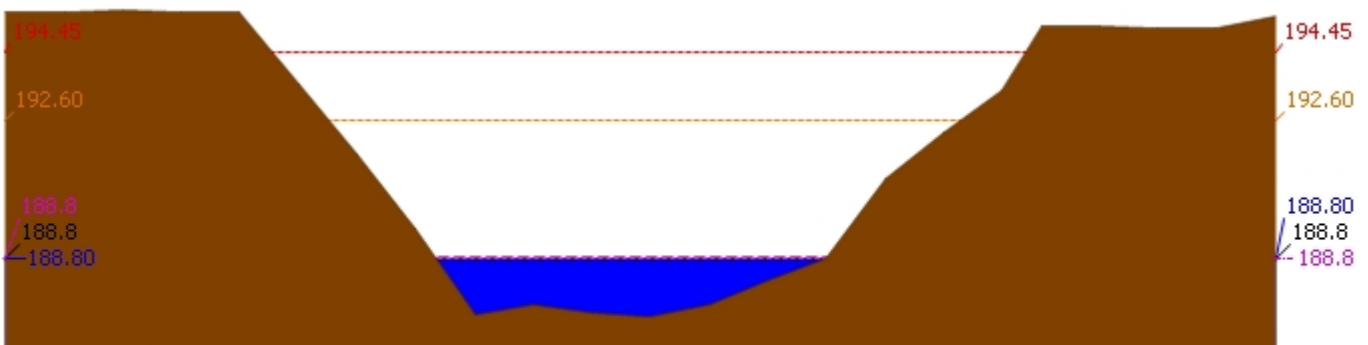
▲ ระดับปัจจุบัน --- ระดับวิกฤติ --- ระดับเฝ้าระวัง ----- เมื่อกาน 7:00 น. - - - - - คาดการณ์ล่วงหน้า 1 วัน สถานี 120901T ห้วยมวกเหล็กที่ อ.มวกเหล็ก ต.มวกเหล็ก อ.มวกเหล็ก จ.สระบุรี ระดับน้ำ 188.80 ม.รทก.
