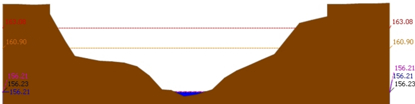
▲ ระดับปัจจุบัน --- ระดับวิกฤติ --- ระดับเฟิาะวัง ---- เมื่อกวาน 7:00 น. - - - - คาคตการล้่วงหน้า 1 วัน สถานี 120105T แม่น้ำป่าสักที่บ้านวังมเหนือ ต.ทำอัญญา อ.หล่มสัก จ.เพชรบูรณ์ ระดับน้ำ 156.21 ม.รทก.
