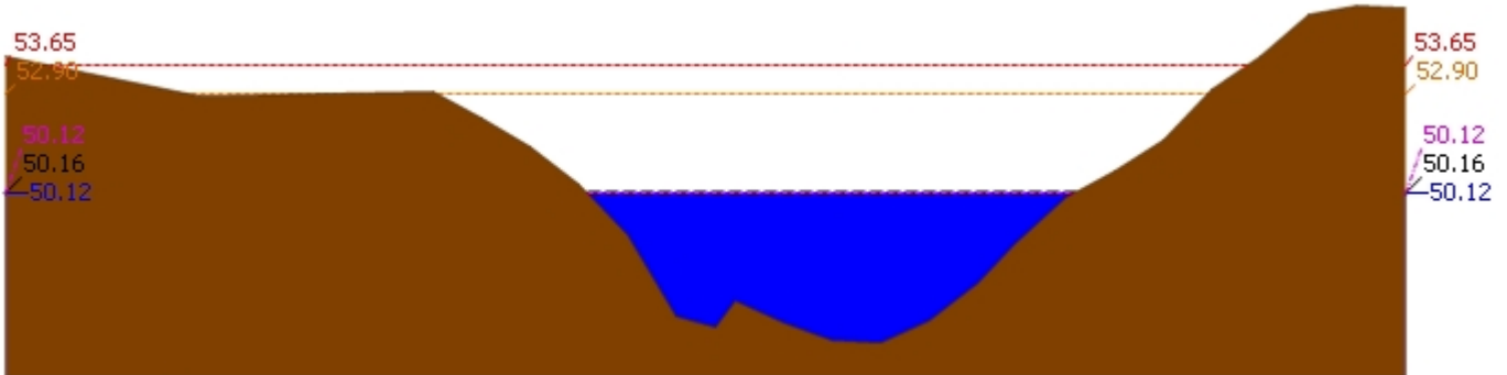
▲ ระดับปัจจุบัน --- ระดับวิกฤติ --- ระดับเฝ้าระวัง ----- เมื่อกาน 7:00 น. - - - - - คาดการณ์ล่วงหน้า 1 วัน สถานี 120113T แม่น้ำป่าสักที่บ้านเขาค้าง ต.คลองกระจิง อ.ศรีเทพ จ.เพชรบูรณ์ ระดับน้ำ 50.12 ม.รทก.
