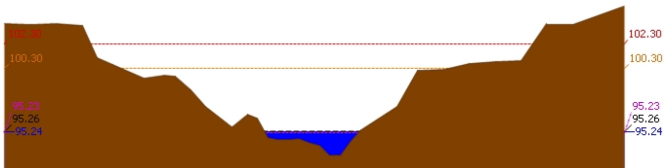
▲ ระดับปัจจุบัน --- ระดับวิกฤติ --- ระดับเฟิาะวัง ---- เมื่อกวาน 7:00 น. - - - - คาคตการล้่วงหน้า 1 วัน สถานี 120112T แม่น้ำป่าสักที่บ้านหนองแหวน ต.วังมะข่อ อ.เมือง จ.เพชรบูรณ์ ระดับน้ำ 95.24 ม.รทก.
