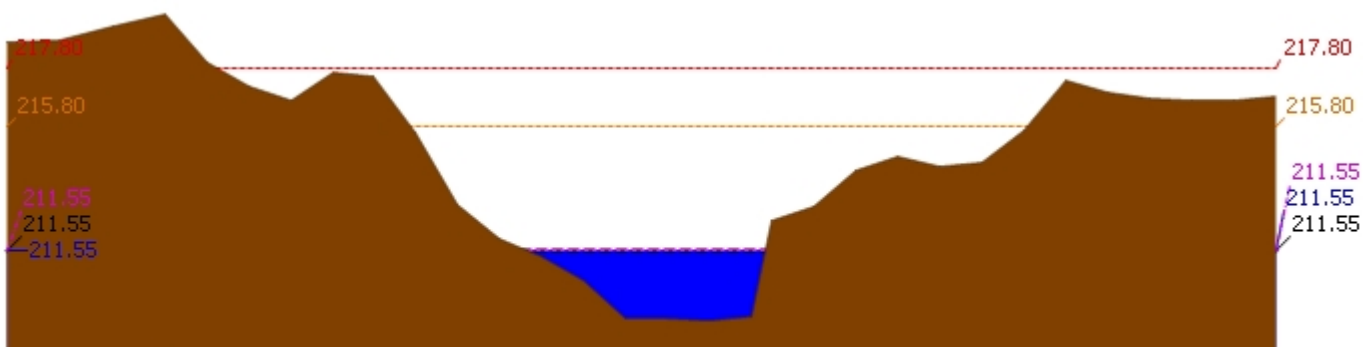
▲ ระดับปัจจุบัน --- ระดับวิกฤติ --- ระดับเฝ้าระวัง ---- เมื่อกวาน 7:00 น. - - - - - คาดการณ์ล่วงหน้า 1 วัน สถานี 120205T แม่น้ำป่าสักที่บ้านอุมกะทาด ต.ศิลา อ.หล่มเก่า จ.เพชรบูรณ์ ระดับน้ำ 211.55 ม.รทก.
