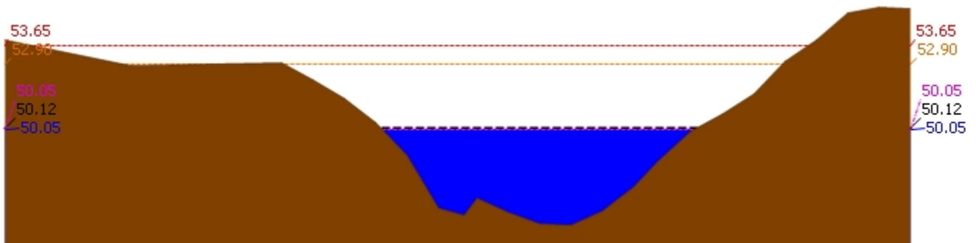
▲ ระดับปัจจุบัน --- ระดับวิกฤติ --- ระดับเฝ้าระวัง ---- เมื่อวาน 7:00 น. - - - - - คาดการณ์ล่วงหน้า 1 วัน สถานี 120113T แม่น้ำป่าสักที่บ้านเขาค้าง ต.คลองกระจิง อ.ศรีเทพ จ.เพชรบูรณ์ ระดับน้ำ 50.05 ม.รทก.
