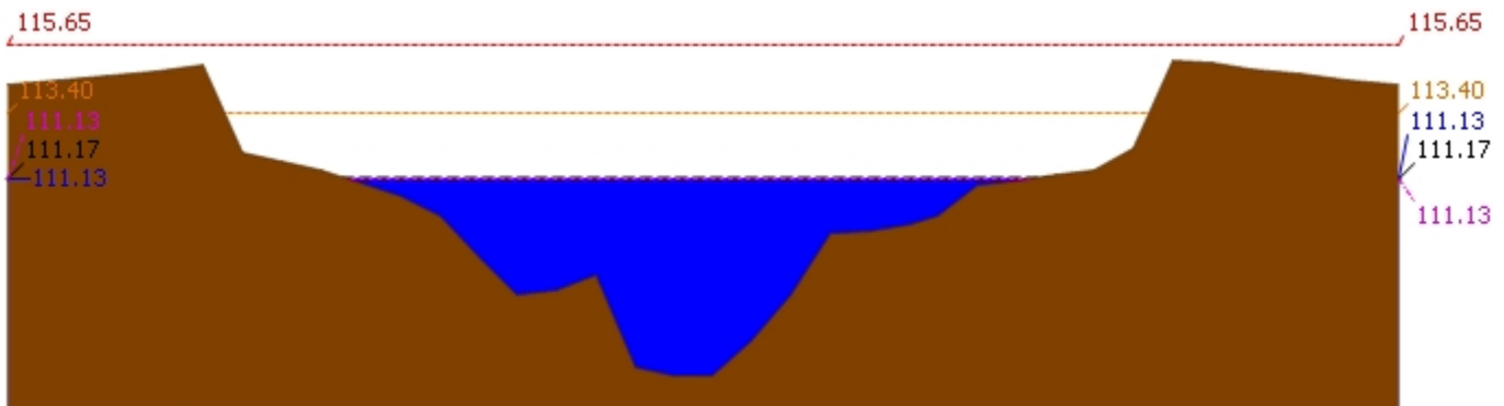
▲ ระดับปัจจุบัน --- ระดับวิกฤติ --- ระดับเฝ้าระวัง ---- เมื่อกวาน 7:00 น. - - - - - คาดการณ์ล่วงหน้า 1 วัน สถานี 120107T แม่น้ำป่าสักที่ อ.เมืองเพชรบูรณ์ ต.นาป่า อ.เมือง จ.เพชรบูรณ์ ระดับน้ำ 111.13 ม.รทก.
