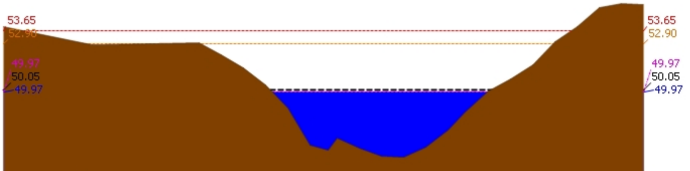
▲ ระดับปัจจุบัน --- ระดับวิกฤติ --- ระดับเฝ้าระวัง ---- เมื่อกว่า 7:00 น. - - - - - คาดการณ์ล่วงหน้า 1 วัน สถานี 120113T แม่น้ำป่าสักที่บ้านเขาค้าง ต.คลองกระจิง อ.ศรีเทพ จ.เพชรบูรณ์ ระดับน้ำ 49.97 ม.รทก.
