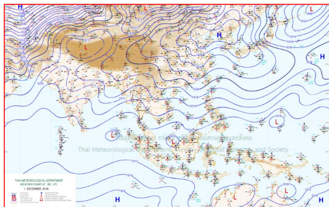
แผนที่อากาศ วันที่ ๑ ธ.ค. ๒๕๖๑ เวลา ๐๗.๐๐ น.
