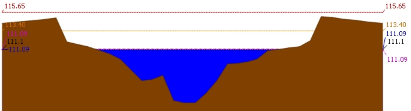
▲ ระดับปัจจุบัน --- ระดับวิกฤติ --- ระดับเฝ้าระวัง ---- เมื่อกวาน 7:00 น. - - - - - คาดการณ์ล่วงหน้า 1 วัน สถานี 120107T แม่น้ำป่าสักที่ อ.เมืองเพชรบูรณ์ ต.นาป่า อ.เมือง จ.เพชรบูรณ์ ระดับน้ำ 111.09 ม.รทก.
