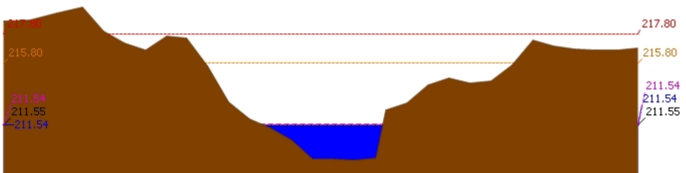
▲ ระดับปัจจุบัน --- ระดับวิกฤติ --- ระดับเฝ้าระวัง ---- เมื่อกวาน 7:00 น. - - - - - คาดการณ์ล่วงหน้า 1 วัน สถานี 120205T แม่น้ำป่าสักที่บ้านอุมกะทาด ต.ศิลา อ.หล่มเก่า จ.เพชรบูรณ์ ระดับน้ำ 211.54 ม.รทก.
