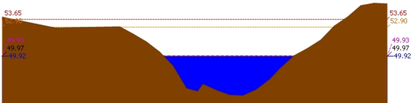
▲ ระดับปัจจุบัน --- ระดับวิกฤติ --- ระดับเฝ้าระวัง ---- เมื่อกาน 7:00 น. - - - - คาดการณ์ล่วงหน้า 1 วัน สถานี 120113T แม่น้ำป่าสักที่บ้านเขาค้าง ต.คลองกระจิง อ.ศรีเทพ จ.เพชรบูรณ์ ระดับน้ำ 49.92 ม.รทก.
