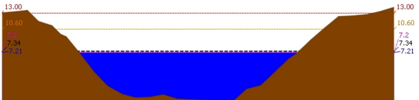
▲ ระดับปัจจุบัน --- ระดับวิกฤติ --- ระดับเฝ้าระวัง ---- เมื่อกวาน 7:00 น. - - - - - คาดการณ์ล่วงหน้า 1 วัน สถานี 120106T แม่น้ำป่าสักที่ อ.เสาไห้ ต.ศาลาวิไทย อ.เสาไห้ จ.สระบุรี ระดับน้ำ 7.21 ม.รทก.
