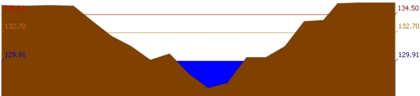
สถานี 120111T แม่น้ำป่าสักที่บ้านจางวาง ต.ลานบัว อ.หล่มสัก จ.เพชรบูรณ์ ระดับน้ำ 129.91 ม.รทก.
