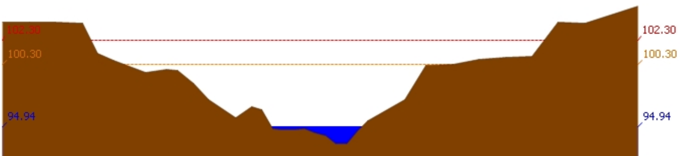
สถานี 120112T แม่น้ำป่าสักที่บ้านหนองแหวน ต.วังมะข่อ อ.เมือง จ.เพชรบูรณ์ ระดับน้ำ 94.94 ม.รทก.
