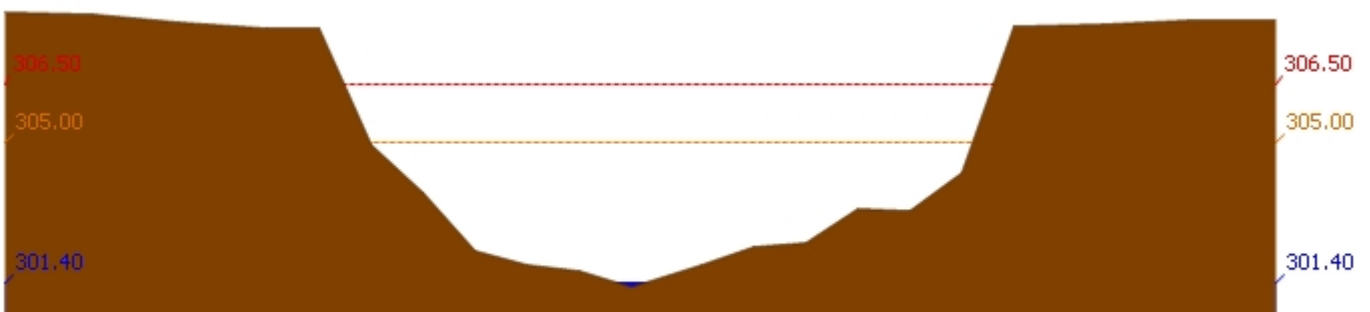
สถานี 120304T ห้วยน้ำพุที่บ้านกกกะบาก ต.โป่ง อ.ด่านซ้าย จ.เลย ระดับน้ำ 301.40 ม.รทก.
