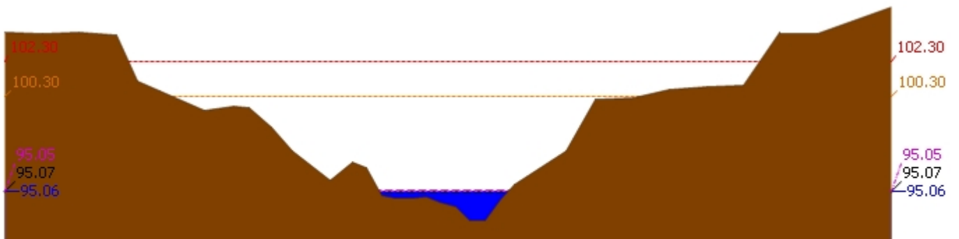
▲ ระดับปัจจุบัน --- ระดับวิกฤติ --- ระดับเฟิาจะวัง ---- เมื่อวาน 7:00 น. ---- คาดการณ์ล่วงหน้า 1 วัน สถานี 120112T แม่น้ำป่าสักที่บ้านหนองแหวน ต.วังมะข่อ อ.เมือง จ.เพชรบูรณ์ ระดับน้ำ 95.06 ม.รทก.
