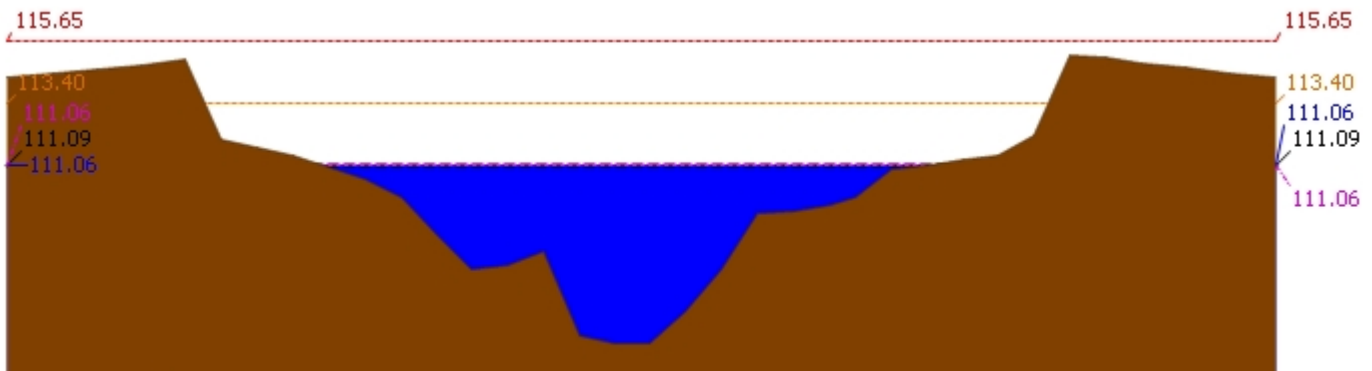
▲ ระดับปัจจุบัน --- ระดับวิกฤติ --- ระดับฝายระวัง ---- เมื่อกาน 7:00 น. - - - - คาคการลลวงหน้า 1 วัน สถานี 120107T แม่น้ำป่าสักที่ อ.เมืองเพชรบูรณ์ ต.นาป่า อ.เมือง จ.เพชรบูรณ์ ระดับน้ำ 111.06 ม.รทก.
