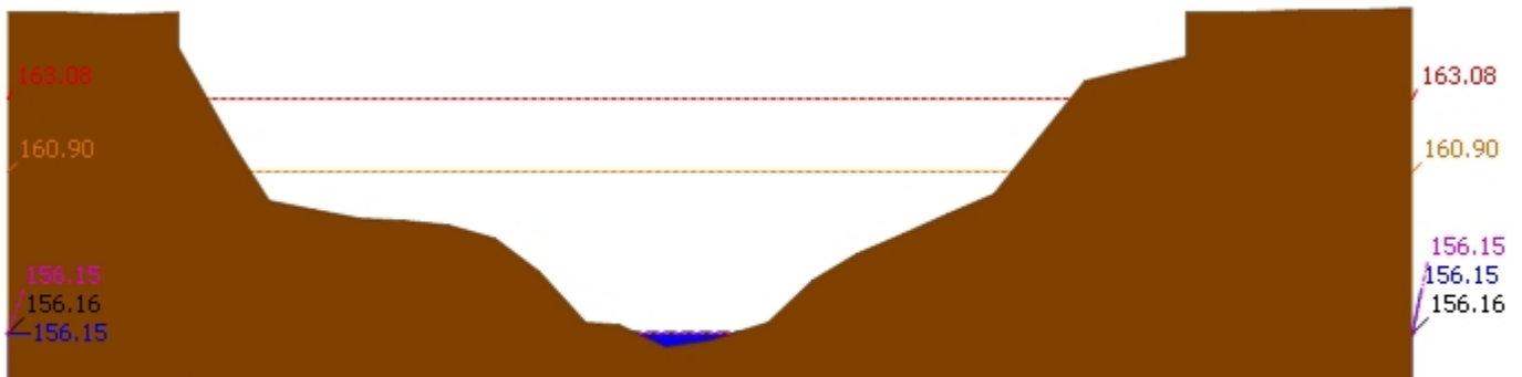
▲ ระดับปัจจุบัน --- ระดับวิกฤติ --- ระดับเฟิาจะวัง ---- เมื่อวาน 7:00 น. ---- คาดการณ์ล่วงหน้า 1 วัน สถานี 120105T แม่น้ำป่าสักที่บ้านวังมเหนื่อ ต.ทำอัญญ อ.หล่มสัก จ.เพชรบูรณ์ ระดับน้ำ 156.15 ม.รทก.
