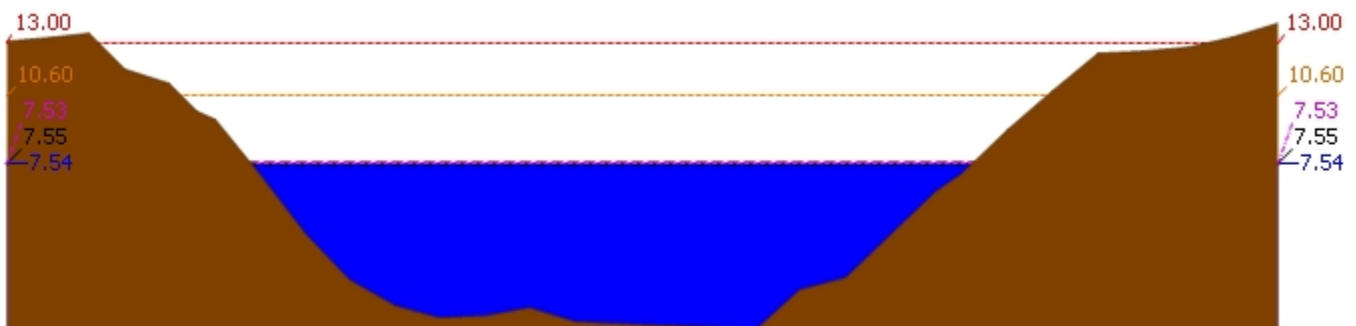
▲ ระดับปัจจุบัน --- ระดับวิกฤติ --- ระดับฝายระวัง ---- เมื่อกาน 7:00 น. - - - - คาคการลลวงหน้า 1 วัน สถานี 120106T แม่น้ำป่าสักที่ อ.เสาไห้ ต.ศาลารีย์ไทย อ.เสาไห้ จ.สระบุรี ระดับน้ำ 7.54 ม.รทก.
