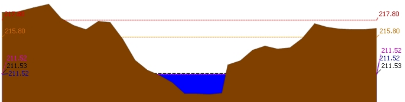
▲ ระดับปัจจุบัน --- ระดับวิกฤติ --- ระดับฝายระวัง ---- เมื่อกาน 7:00 น. - - - - คาคการลลวงหน้า 1 วัน สถานี 120205T แม่น้ำป่าสักที่บ้านอุมกะทาด ต.ศิลา อ.หล่มเก่า จ.เพชรบูรณ์ ระดับน้ำ 211.52 ม.รทก.
