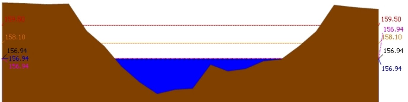
▲ ระดับปัจจุบัน --- ระดับวิกฤติ --- ระดับเฟิาจะวัง ---- เมื่อวาน 7:00 น. ---- คาดการณ์ล่วงหน้า 1 วัน สถานี 120305T หัวน้ำพุทที่ อ.หล่มเก่า ต.หล่มเก่า อ.หล่มเก่า จ.เพชรบูรณ์ ระดับน้ำ 156.94 ม.รทก.
