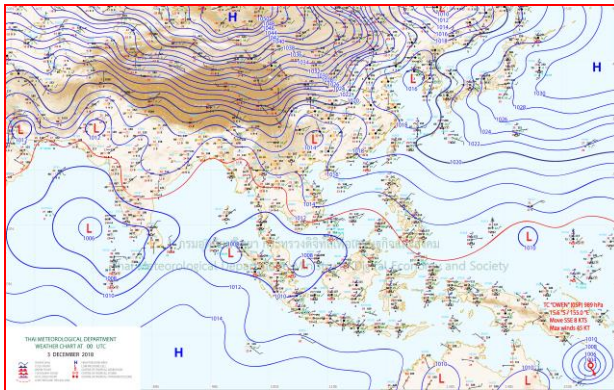
แผนที่อากาศ วันที่ 3 ธ.ค. 2561 เวลา 07.00 น. ภาพถ่ายจากดาวเทียม วันที่ 3 ธ.ค. 2561
