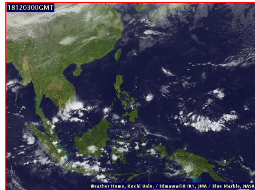
แผนที่อากาศ วันที่ 3 ธ.ค. 2561 เวลา 07.00 น. ภาพถ่ายจากดาวเทียม วันที่ 3 ธ.ค. 2561
