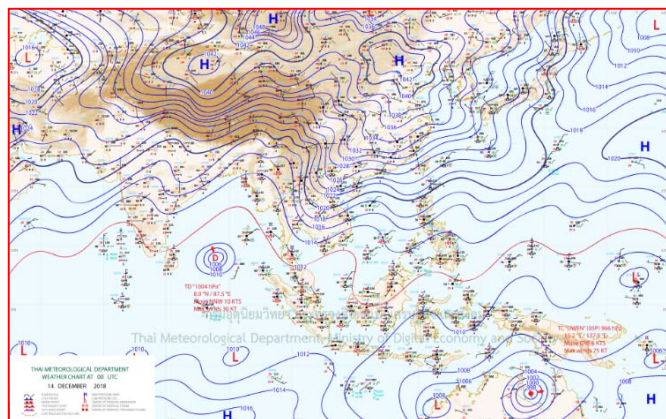
แผนที่อากาศ วันที่ ๑๔ ธ.ค.๒๕๖๑ เวลา ๐๗.๐๐น.
