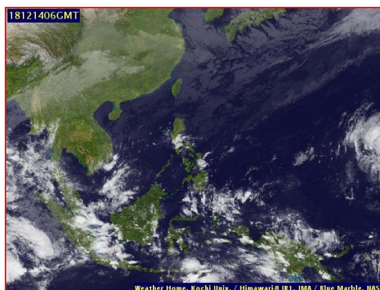
ภาพถ่ายดาวเทียม วันที่ ๑๔ ธ.ค. ๒๕๖๑ เวลา ๑๓.๐๐น.
