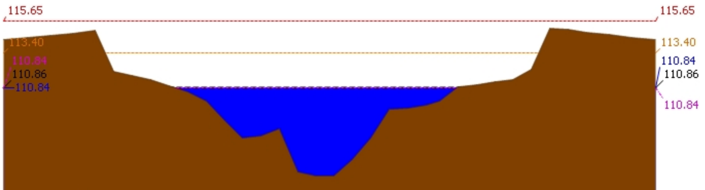
▲ ระดับปัจจุบัน --- ระดับวิกฤติ --- ระดับเฟิาระวัง ---- เมื่อวาน 7:00 น. - - - - คาคตการลลวงหน้า 1 วัน สถานี 120107T แม่น้ำป่าสักที่ อ.เมืองเพชรบูรณ์ ต.นาป่า อ.เมือง จ.เพชรบูรณ์ ระดับน้ำ 110.84 ม.รทก.
