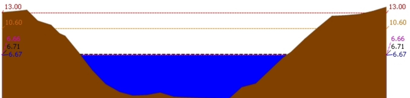
▲ ระดับปัจจุบัน --- ระดับวิกฤติ --- ระดับเฟิาระวัง ---- เมื่อวาน 7:00 น. - - - - คาคตการลลวงหน้า 1 วัน สถานี 120106T แม่น้ำป่าสักที่ อ.เสาไห้ ต.ศาลาริไทย อ.เสาไห้ จ.สระบุรี ระดับน้ำ 6.67 ม.รทก.
