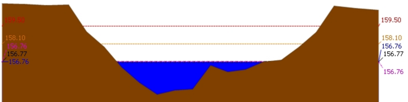
▲ ระดับปัจจุบัน --- ระดับวิกฤติ --- ระดับเฝ้าระวัง ---- เมื่อวาน 7:00 น. - - - - - คาดการณ์ล่วงหน้า 1 วัน สถานี 120305T หัวน้ำพุที่ อ.หล่มเก่า ต.หล่มเก่า อ.หล่มเก่า จ.เพชรบูรณ์ ระดับน้ำ 156.76 ม.รทก.
