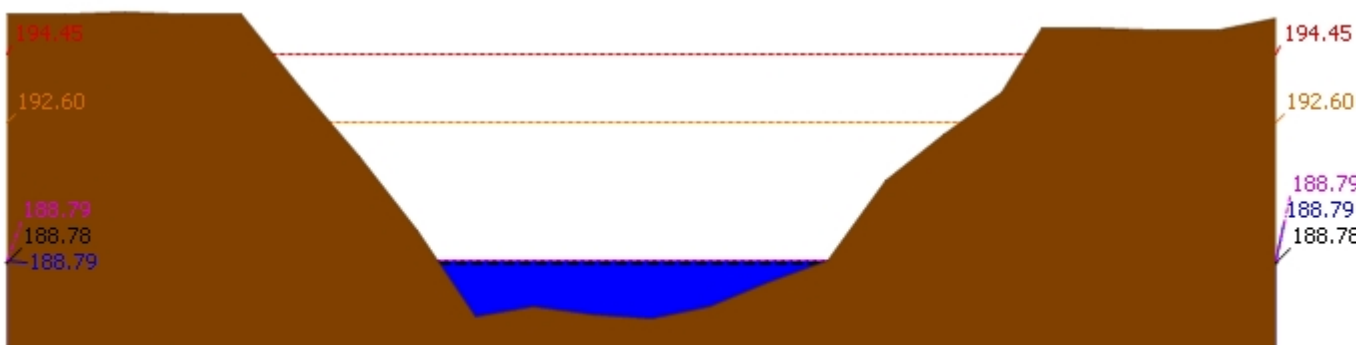
▲ ระดับปัจจุบัน --- ระดับวิกฤติ --- ระดับเฝ้าระวัง ---- เมื่อกวาน 7:00 น. - - - - - คาดการณ์ล่วงหน้า 1 วัน สถานี 120901T ห้วยมวกเหล็กที่ อ.มวกเหล็ก ต.มวกเหล็ก อ.มวกเหล็ก จ.สระบุรี ระดับน้ำ 188.79 ม.รทก.
