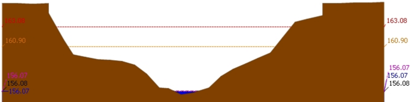
▲ ระดับปัจจุบัน --- ระดับวิกฤติ --- ระดับเฝ้าระวัง ---- เมื่อวาน 7:00 น. - - - - - คาดการณ์ล่วงหน้า 1 วัน สถานี 120105T แม่น้ำป่าสักที่บ้านวังมเหนื่อ ต.ทำอัญญา อ.หล่มสัก จ.เพชรบูรณ์ ระดับน้ำ 156.07 ม.รทก.
