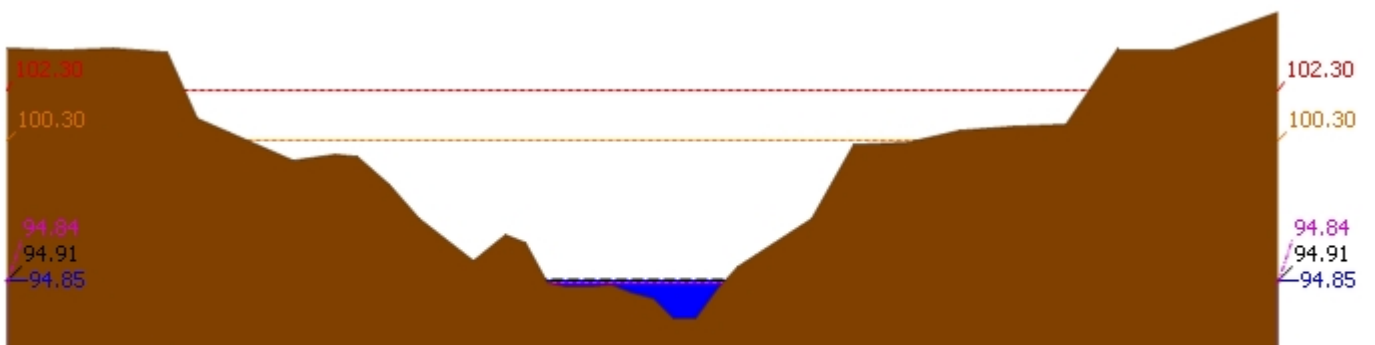
▲ ระดับปัจจุบัน --- ระดับวิกฤติ --- ระดับเฝ้าระวัง ---- เมื่อวาน 7:00 น. - - - - - คาดการณ์ล่วงหน้า 1 วัน สถานี 120112T แม่น้ำป่าสักที่บ้านหนองแหวน ต.วังมะข่อ อ.เมือง จ.เพชรบูรณ์ ระดับน้ำ 94.85 ม.รทก.
