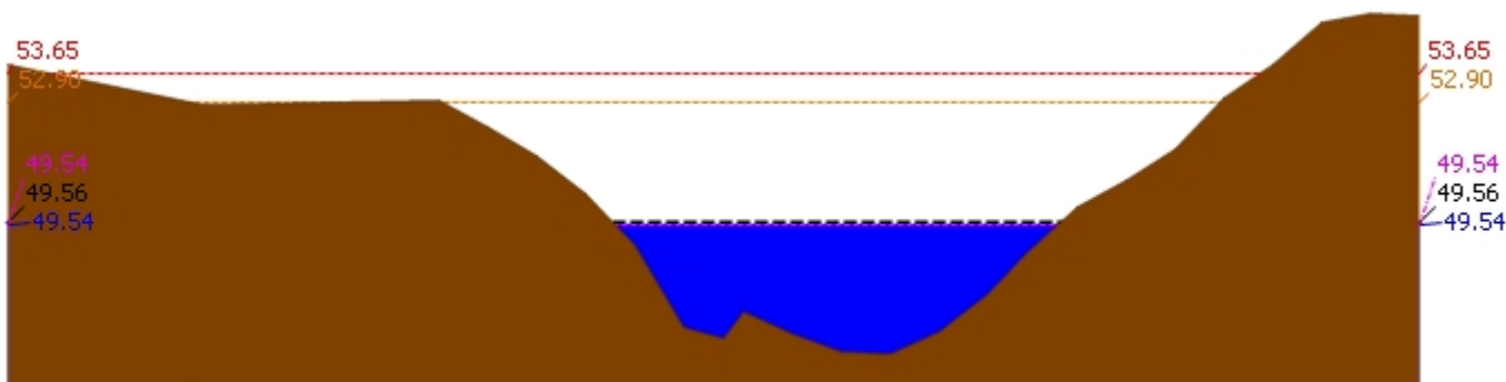
▲ ระดับปัจจุบัน --- ระดับวิกฤติ --- ระดับเฝ้าระวัง ---- เมื่อกวาน 7:00 น. - - - - - คาดการณ์ล่วงหน้า 1 วัน สถานี 120113T แม่น้ำป่าสักที่บ้านเขาค้าง ต.คลองกระจิง อ.ศรีเทพ จ.เพชรบูรณ์ ระดับน้ำ 49.54 ม.รทก.
