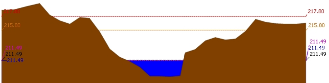
▲ ระดับปัจจุบัน --- ระดับวิกฤติ --- ระดับเฟิาระวัง ---- เมื่อกาน 7:00 น. - - - - คาคการล่ลวงหน้า 1 วัน สถานี 120205T แม่น้ำป่าสักที่ บ้านอู่กะทาด ต.ศิลา อ.หล่มเก่า จ.เพชรบูรณ์ ระดับน้ำ 211.49 ม.รทก.
