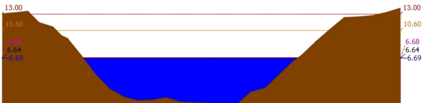
▲ ระดับปัจจุบัน --- ระดับวิกฤติ --- ระดับเฟิาระวัง ---- เมื่อกาน 7:00 น. - - - - คาคการล่ลวงหน้า 1 วัน สถานี 120106T แม่น้ำป่าสักที่ อ.เสาไห้ ต.ศาลาริไทย อ.เสาไห้ จ.สระบุรี ระดับน้ำ 6.69 ม.รทก.
