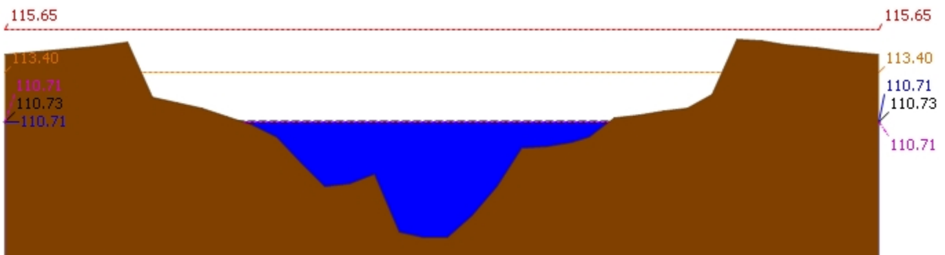
▲ ระดับปัจจุบัน --- ระดับวิกฤติ --- ระดับเฟิาระวัง ---- เมื่อกาน 7:00 น. - - - - คาคการล่ลวงหน้า 1 วัน สถานี 120107T แม่น้ำป่าสักที่ อ.เมืองเพชรบูรณ์ ต.นาป่า อ.เมือง จ.เพชรบูรณ์ ระดับน้ำ 110.71 ม.รทก.
