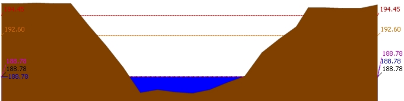
▲ ระดับปัจจุบัน --- ระดับวิกฤติ --- ระดับฝายระวัง ---- เมื่อวาน 7:00 น. - - - - - คาดการณ์ล่วงหน้า 1 วัน สถานี 120901T ห้วยมวกเหล็กที่ อ.มวกเหล็ก ต.มวกเหล็ก อ.มวกเหล็ก จ.สระบุรี ระดับน้ำ 188.78 ม.รทก.
