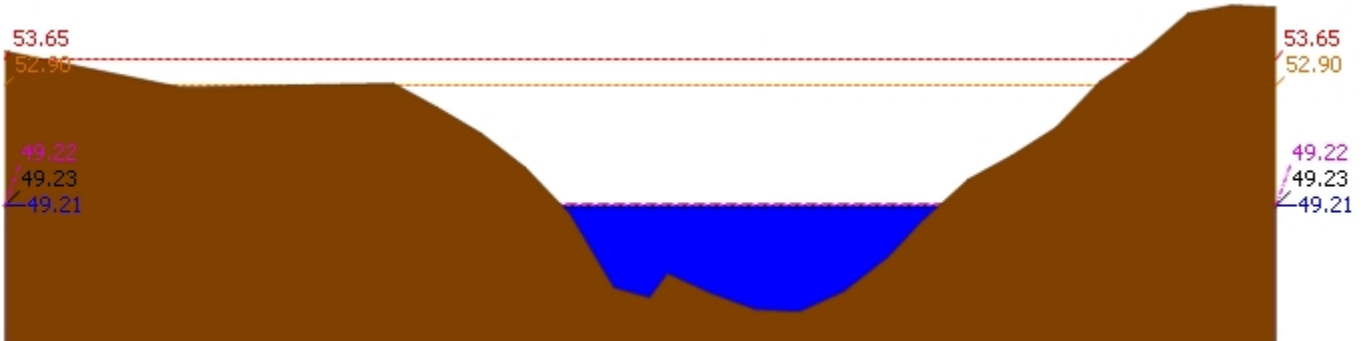
▲ ระดับปัจจุบัน --- ระดับวิกฤติ --- ระดับฝายระวัง ---- เมื่อวาน 7:00 น. - - - - - คาดการณ์ล่วงหน้า 1 วัน สถานี 120113T แม่น้ำป่าสักที่บ้านเขาค้าง ต.คลองกระจิง อ.ศรีเทพ จ.เพชรบูรณ์ ระดับน้ำ 49.21 ม.รทก.
