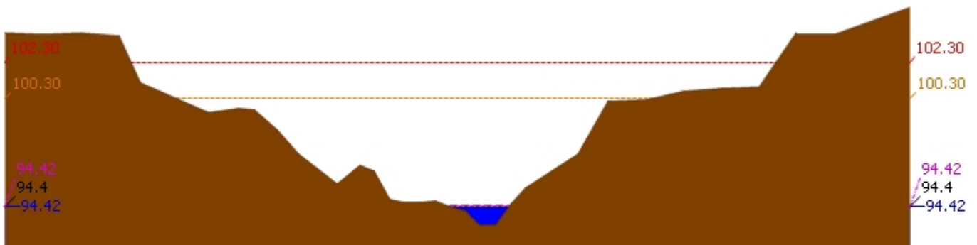
▲ ระดับปัจจุบัน --- ระดับวิกฤติ --- ระดับเฝ้าระวัง ---- เมื่อวาน 7:00 น. - - - - - คาดการณ์ล่วงหน้า 1 วัน สถานี 120112T แม่น้ำป่าสักที่บ้านหนองแหวน ต.วังมะข่อ อ.เมือง จ.เพชรบูรณ์ ระดับน้ำ 94.42 ม.รทก.
