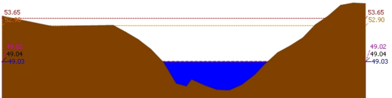
▲ ระดับปัจจุบัน --- ระดับวิกฤติ --- ระดับเฝ้าระวัง ---- เมื่อกวาน 7:00 น. - - - - คาดการณ์ล่วงหน้า 1 วัน สถานี 120113T แม่น้ำป่าสักที่บ้านเขาค้าง ต.คลองกระจิง อ.ศรีเทพ จ.เพชรบูรณ์ ระดับน้ำ 49.03 ม.รทก.
