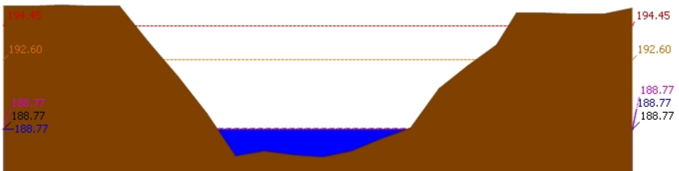
▲ ระดับปัจจุบัน --- ระดับวิกฤติ --- ระดับเฝ้าระวัง ---- เมื่อกวาน 7:00 น. - - - - คาดการณ์ล่วงหน้า 1 วัน สถานี 120901T ห้วยมวกเหล็กที่ อ.มวกเหล็ก ต.มวกเหล็ก อ.มวกเหล็ก จ.สระบุรี ระดับน้ำ 188.77 ม.รทก.
