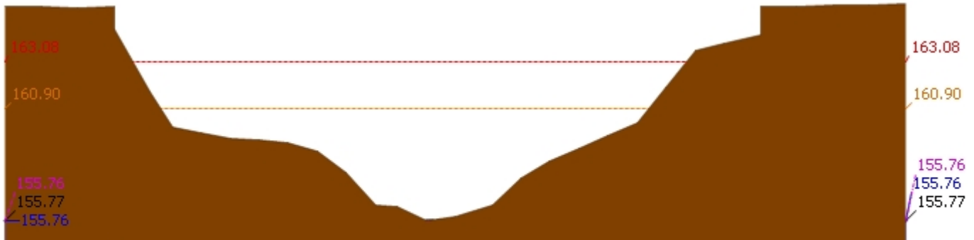
▲ ระดับปัจจุบัน --- ระดับวิกฤติ --- ระดับเฝ้าระวัง ---- เมื่อวาน 7:00 น. - - - - - คาดการณ์ล่วงหน้า 1 วัน สถานี 120105T แม่น้ำป่าสักที่บ้านวังมเสหนือ ต.ทำอัญญา อ.หล่มสัก จ.เพชรบูรณ์ ระดับน้ำ 155.76 ม.รทก.
