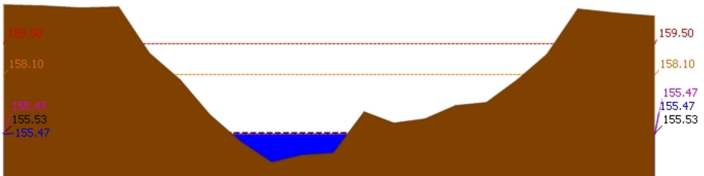
▲ ระดับปัจจุบัน --- ระดับวิกฤติ --- ระดับเฝ้าระวัง ---- เมื่อวาน 7:00 น. - - - - - คาดการณ์ล่วงหน้า 1 วัน สถานี 120305T หัวน้ำพุอยู่ที่ อ.หล่มเก่า ต.หล่มเก่า อ.หล่มเก่า จ.เพชรบูรณ์ ระดับน้ำ 155.47 ม.รทก.
