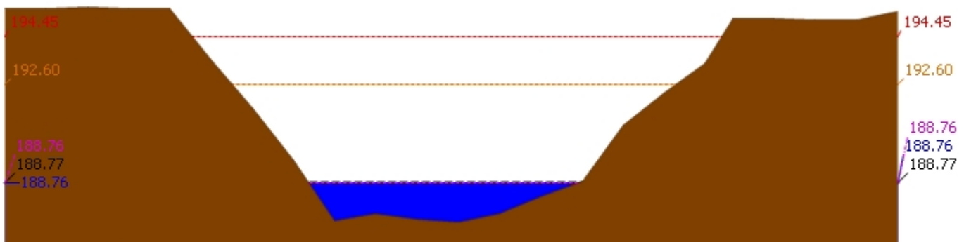
▲ ระดับปัจจุบัน --- ระดับวิกฤติ --- ระดับฝายระวัง ---- เมื่อวาน 7:00 น. - - - - - คาดการณ์ล่วงหน้า 1 วัน สถานี 120901T ห้วยมวกเหล็กที่ อ.มวกเหล็ก ต.มวกเหล็ก อ.มวกเหล็ก จ.สระบุรี ระดับน้ำ 188.76 ม.รทก.
