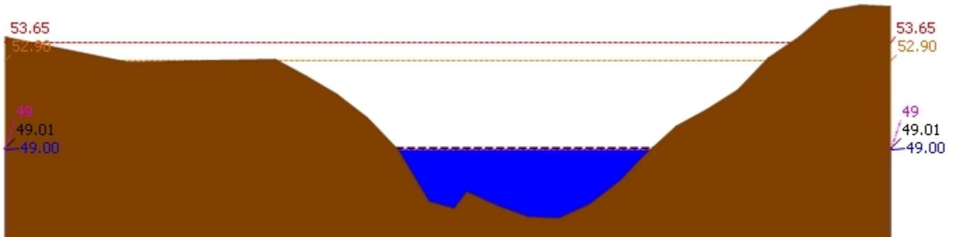
▲ ระดับปัจจุบัน --- ระดับวิกฤติ --- ระดับฝายระวัง ---- เมื่อวาน 7:00 น. - - - - - คาดการณ์ล่วงหน้า 1 วัน สถานี 120113T แม่น้ำป่าสักที่บ้านเขาค้าง ต.คลองกระจิง อ.ศรีเทพ จ.เพชรบูรณ์ ระดับน้ำ 49.00 ม.รทก.
