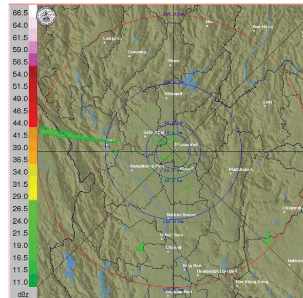
ภาพเรดาร์ตรวจอากาศ "พิชฌุโลก" ณ วันที่ 24 มกราคม 2562 (ที่มา : กรมอุตุนิยมวิทยา)
