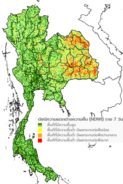
แผนที่ดาวเทียมของ Gistda (18 - 24 ม.ค.62)
