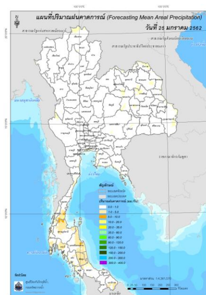
ปริมาณฝนคาดการณ์ในวันที่ 25 มกราคม 2562
