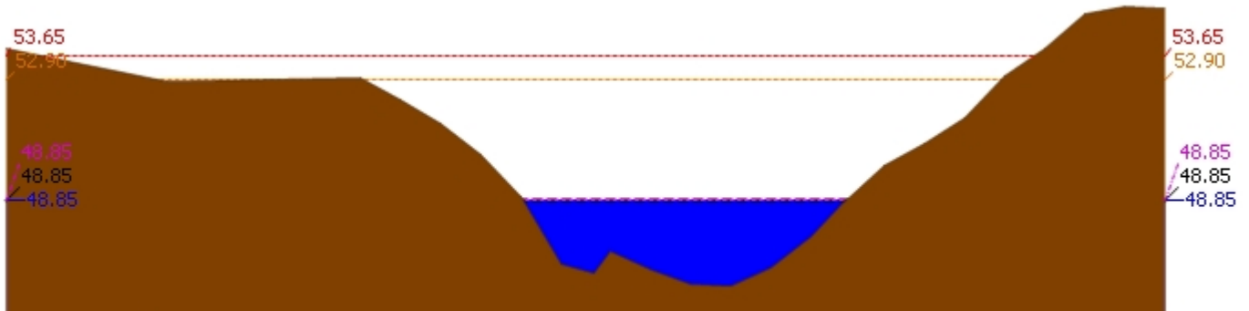
▲ ระดับปัจจุบัน --- ระดับวิกฤติ --- ระดับเฝ้าระวัง ---- เมื่อวาน 7:00 น. - - - - - คาดการณ์ล่วงหน้า 1 วัน สถานี 120113T แม่น้ำป่าสักที่บ้านเขาค้าง ต.คลองกระจิง อ.ศรีเทพ จ.เพชรบูรณ์ ระดับน้ำ 48.85 ม.รทก.
