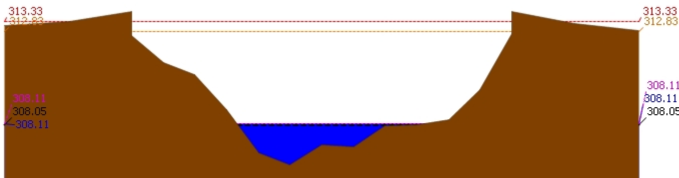
▲ ระดับปัจจุบัน --- ระดับวิกฤติ --- ระดับฝายระวัง ---- เมื่อกวาน 7:00 น. - - - - - คาดการณ์ล่วงหน้า 1 วัน สถานี 060814T น้ำแม่ฆานที่บ้านท่าโป่ง ต.บ้านแม อ.สันป่าตอง จ.เชียงใหม่ ระดับน้ำ 308.11 ม.รทก.
