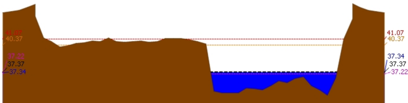
▲ ระดับปัจจุบัน --- ระดับวิกฤติ --- ระดับฝายระวัง ---- เมื่อกวาน 7:00 น. - - - - - คาดการณ์ล่วงหน้า 1 วัน สถานี 060110T แม่น้ำปิงที่บ้านบางแก้ว ต.บางแก้ว อ.บรรพตพิสัย จ.นครสวรรค์ ระดับน้ำ 37.34 ม.รทก.
