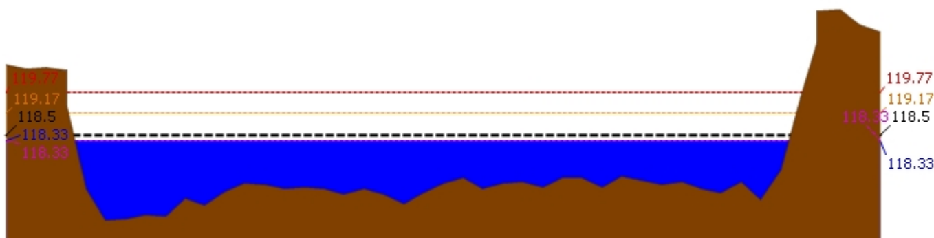
▲ ระดับปัจจุบัน --- ระดับวิกฤติ --- ระดับฝายระวัง ---- เมื่อกวาน 7:00 น. - - - - - คาดการณ์ล่วงหน้า 1 วัน สถานี 060111T แม่น้ำปิงที่บ้านปากร่องห้วยจี่ ต.ตากออก อ.บ้านตาก จ.ตาก ระดับน้ำ 118.33 ม.รทก.
