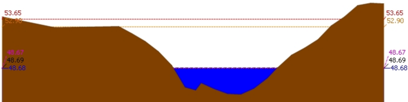
▲ ระดับปัจจุบัน --- ระดับวิกฤติ --- ระดับฝายระวัง ----- เมื่อวาน 7:00 น. - - - - - คาดการณ์ล่วงหน้า 1 วัน สถานี 120113T แม่น้ำป่าสักที่บ้านเขาค้าง ต.คลองกระจิง อ.ศรีเทพ จ.เพชรบูรณ์ ระดับน้ำ 48.68 ม.รทก.
