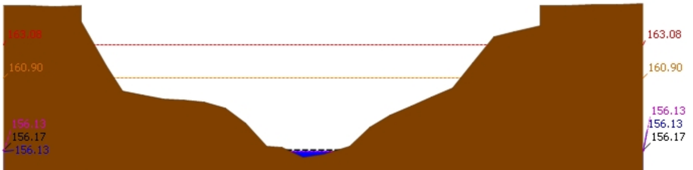
▲ ระดับปัจจุบัน --- ระดับวิกฤติ --- ระดับฝายระวัง ---- เมื่อวาน 7:00 น. - - - - - คาดการณ์ล่วงหน้า 1 วัน สถานี 120105T แม่น้ำป่าสักที่บ้านวังมเหนื่อ ต.ทำอัญญ อ.หล่มสัก จ.เพชรบูรณ์ ระดับน้ำ 156.13 ม.รทก.
