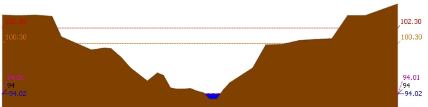
▲ ระดับปัจจุบัน --- ระดับวิกฤติ --- ระดับฝายระวัง ---- เมื่อวาน 7:00 น. - - - - - คาดการณ์ล่วงหน้า 1 วัน สถานี 120112T แม่น้ำป่าสักที่บ้านหนองแหวน ต.วังมะข่อ อ.เมือง จ.เพชรบูรณ์ ระดับน้ำ 94.02 ม.รทก.
