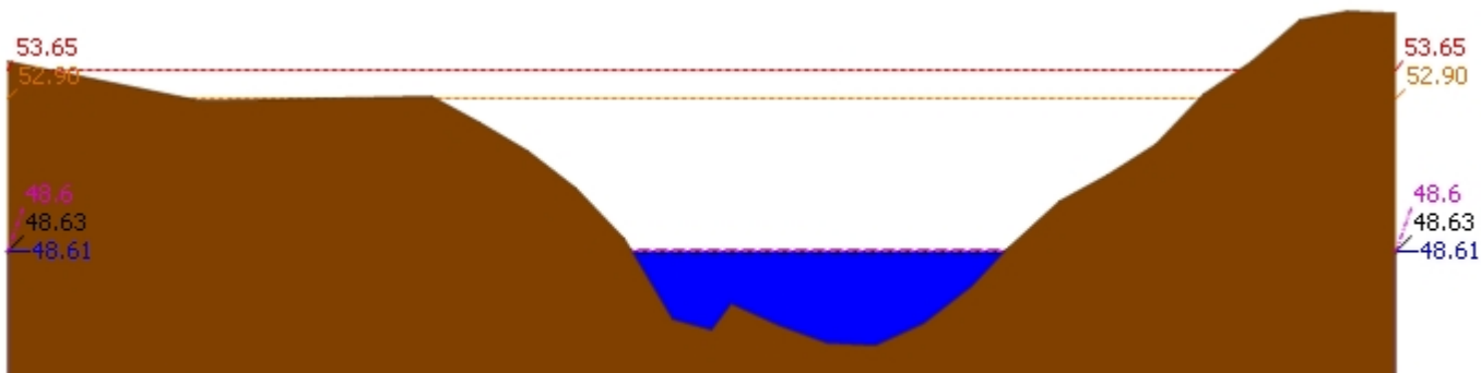
▲ ระดับปัจจุบัน --- ระดับวิกฤติ --- ระดับเฝ้าระวัง ---- เมื่อกวาน 7:00 น. - - - - คาดการณ์ล่วงหน้า 1 วัน สถานี 120113T แม่น้ำป่าสักที่บ้านเขาค้าง ต.คลองกระดัง อ.ศรีเทพ จ.เพชรบูรณ์ ระดับน้ำ 48.61 ม.รทก.
