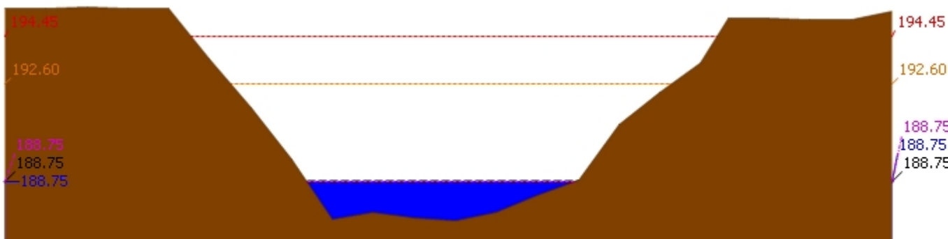
▲ ระดับปัจจุบัน --- ระดับวิกฤติ --- ระดับเฝ้าระวัง ---- เมื่อกวาน 7:00 น. - - - - คาดการณ์ล่วงหน้า 1 วัน สถานี 120901T ห้วยมวกเหล็กที่ อ.มวกเหล็ก ต.มวกเหล็ก อ.มวกเหล็ก จ.สระบุรี ระดับน้ำ 188.75 ม.รทก.
