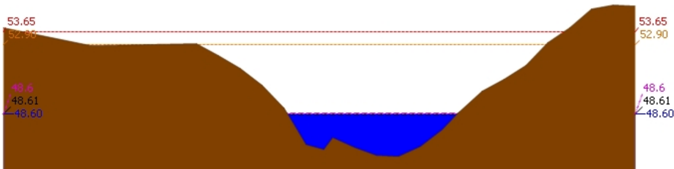
▲ ระดับปัจจุบัน --- ระดับวิกฤติ --- ระดับเฝ้าระวัง ---- เมื่อกวาน 7:00 น. - - - - คาดการณ์ล่วงหน้า 1 วัน สถานี 120113T แม่น้ำป่าสักที่บ้านเขาค้าง ต.คลองกระจิง อ.ศรีเทพ จ.เพชรบูรณ์ ระดับน้ำ 48.60 ม.รทก.
