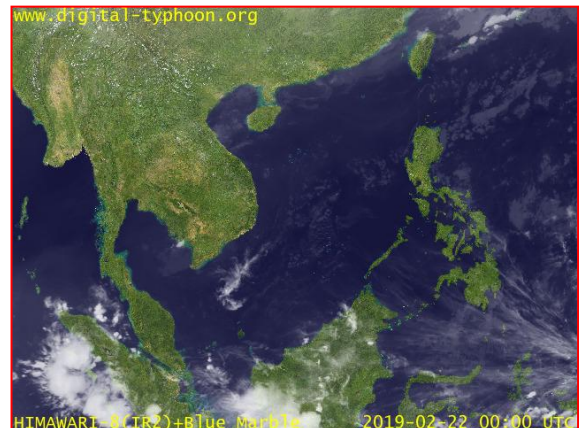
ภาพถ่ายจากดาวเทียม วันที่ 22 ก.พ. 2562
