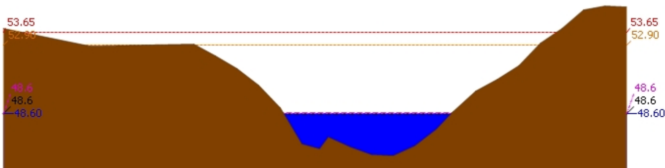
▲ ระดับปัจจุบัน --- ระดับวิกฤติ --- ระดับเฝ้าระวัง ---- เมื่อวาน 7:00 น. - - - - - คาดการณ์ล่วงหน้า 1 วัน สถานี 120113T แม่น้ำป่าสักที่บ้านเขาค้าง ต.คลองกระดังง์ อ.ศรีเทพ จ.เพชรบูรณ์ ระดับน้ำ 48.60 ม.รทก.
