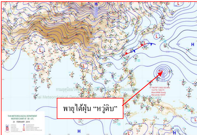
แผนที่อากาศ วันที่ ๒๕ ก.พ. ๒๕๖๒ เวลา ๐๗.๐๐ น.
