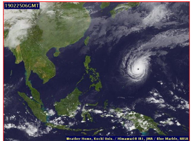
ภาพถ่ายดาวเทียม วันที่ ๒๕ ก.พ. ๒๕๖๒ เวลา ๑๓.๐๐ น.
