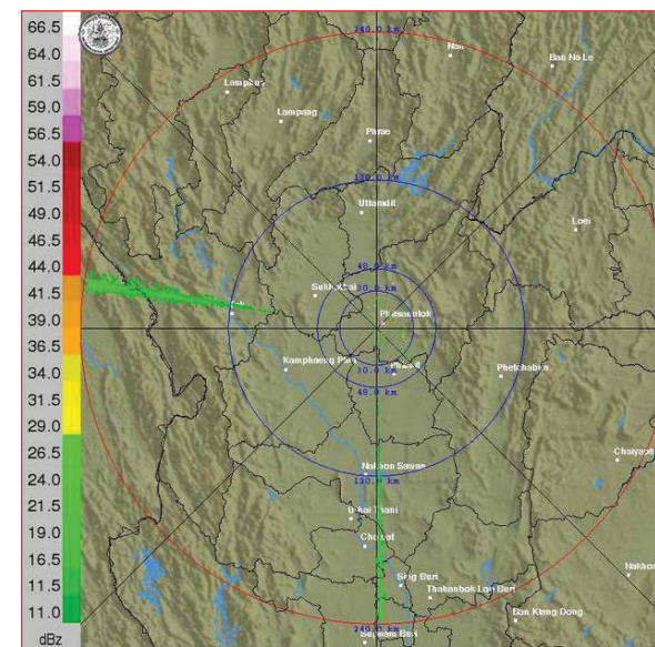
ภาพเรดาร์ตรวจอากาศ "พิษณุโลก" ณ วันที่ 25 กุมภาพันธ์ 2562 (ที่มา : กรมอุตุนิยมวิทยา)
