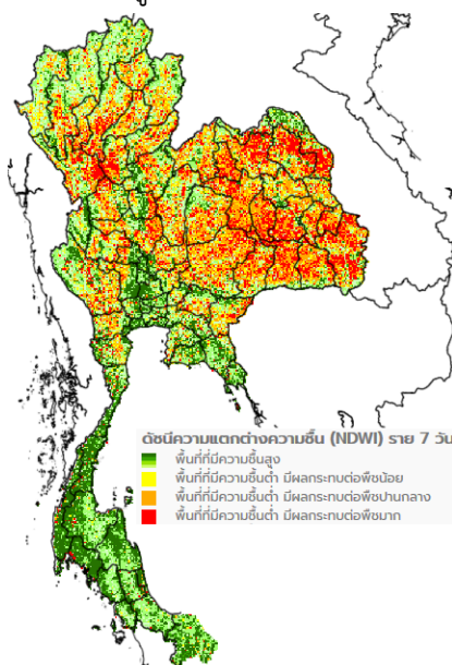
แผนที่ดาวเทียมของ Gistda (19 - 25 ก.พ.62)
