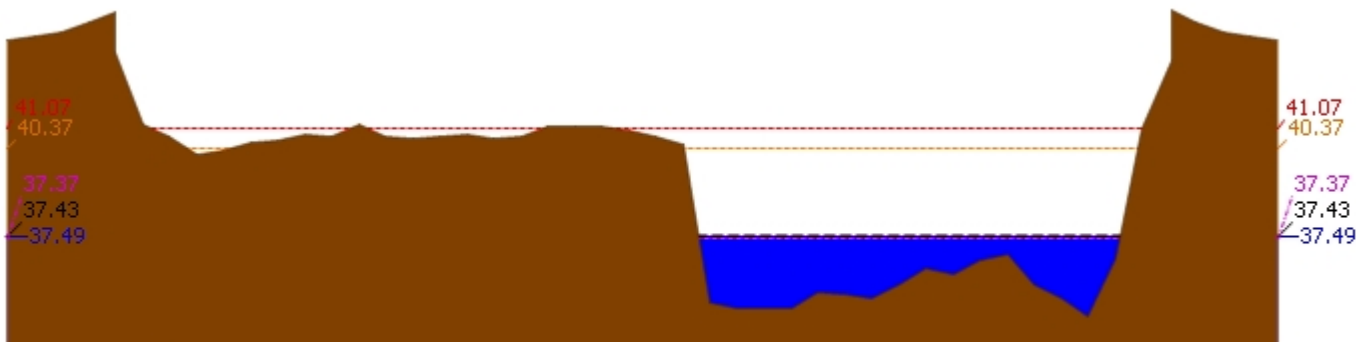
▲ ระดับปัจจุบัน --- ระดับวิกฤติ --- ระดับเฝ้าระวัง ---- เมื่อวาน 7:00 น. - - - - - คาดการณ์ล่วงหน้า 1 วัน สถานี 060110T แม่น้ำปิงที่บ้านบางแก้ว ต.บางแก้ว อ.บรรพตพิสัย จ.นครสวรรค์ ระดับน้ำ 37.49 ม.รทก.
