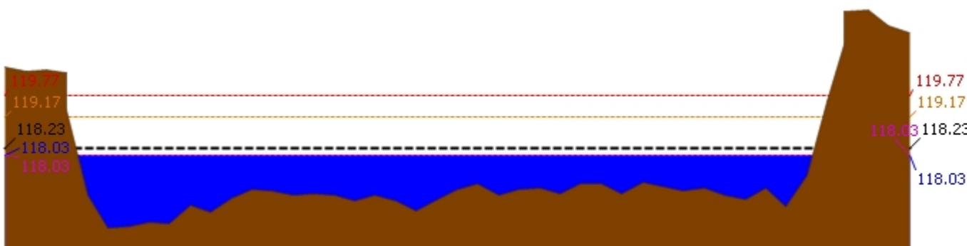
▲ ระดับปัจจุบัน --- ระดับวิกฤติ --- ระดับเฝ้าระวัง ---- เมื่อวาน 7:00 น. - - - - - คาดการณ์ล่วงหน้า 1 วัน สถานี 060111T แม่น้ำปิงที่บ้านปากร่องห้วยจี่ ต.ตากออก อ.บ้านตาก จ.ตาก ระดับน้ำ 118.03 ม.รทก.
