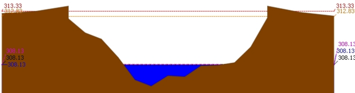
▲ ระดับปัจจุบัน --- ระดับวิกฤติ --- ระดับเฝ้าระวัง ---- เมื่อวาน 7:00 น. - - - - - คาดการณ์ล่วงหน้า 1 วัน สถานี 060814T น้ำแม่ขานที่บ้านท่าโป่ง ต.บ้านแม อ.สันป่าตอง จ.เชียงใหม่ ระดับน้ำ 308.13 ม.รทก.
