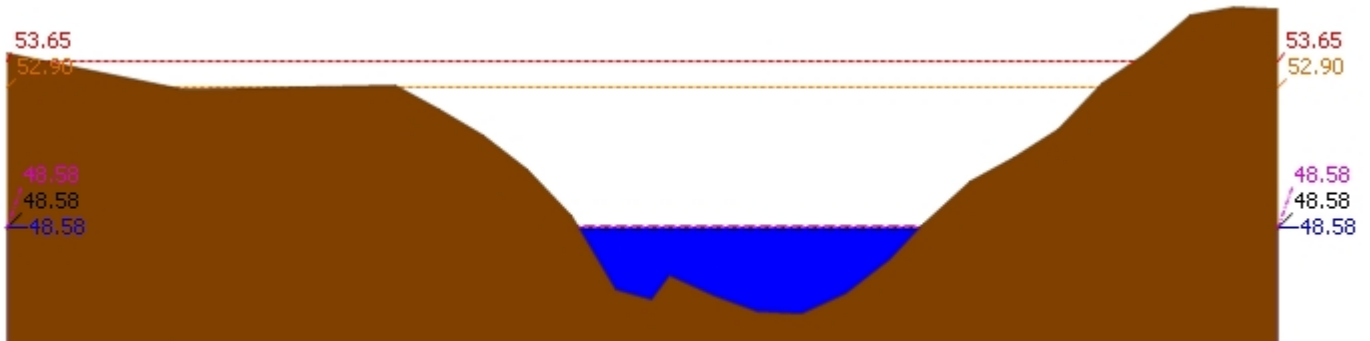
▲ ระดับปัจจุบัน --- ระดับวิกฤติ --- ระดับเฝ้าระวัง ---- เมื่อวาน 7:00 น. - - - - - คาดการณ์ล่วงหน้า 1 วัน สถานี 120113T แม่น้ำป่าสักที่บ้านเขาค้าง ต.คลองกระจิง อ.ศรีเทพ จ.เพชรบูรณ์ ระดับน้ำ 48.58 ม.รทก.
