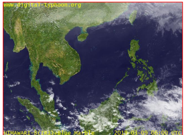
ภาพถ่ายดาวเทียม วันที่ ๙ มี.ค. ๒๕๖๒ เวลา ๑๓.๐๐ น.
