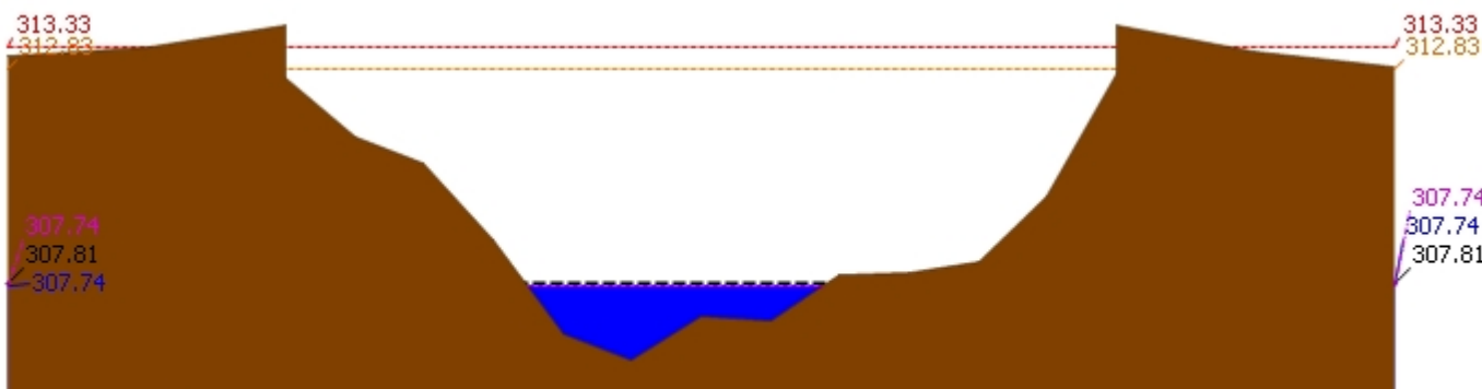
▲ ระดับปัจจุบัน --- ระดับวิกฤติ --- ระดับฝายระวัง ---- เมื่อกวาน 7:00 น. --- คาดการณ์ล่วงหน้า 1 วัน สถานี 060814T น้ำแม่ขานที่บ้านท่าโป่ง ต.บ้านแม อ.สันป่าตอง จ.เชียงใหม่ ระดับน้ำ 307.74 ม.รทก.
