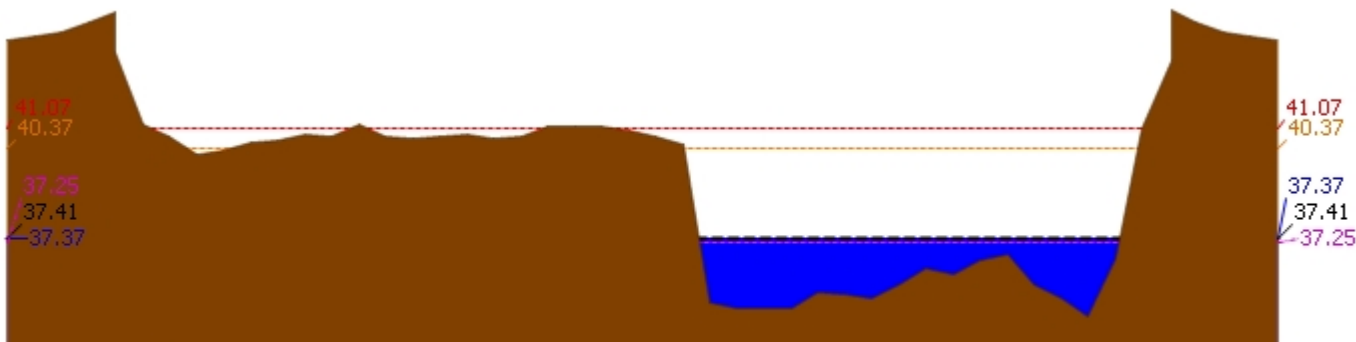
▲ ระดับปัจจุบัน --- ระดับวิกฤติ --- ระดับฝายระวัง ---- เมื่อกวาน 7:00 น. --- คาดการณ์ล่วงหน้า 1 วัน สถานี 060110T แม่น้ำปิงที่บ้านบางแก้ว ต.บางแก้ว อ.บรรพตพิสัย จ.นครสวรรค์ ระดับน้ำ 37.37 ม.รทก.
