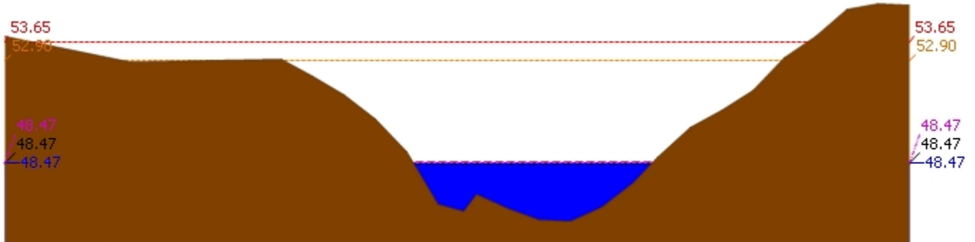
▲ ระดับปัจจุบัน --- ระดับวิกฤติ --- ระดับเฝ้าระวัง ---- เมื่อวาน 7:00 น. - - - - - คาดการณ์ล่วงหน้า 1 วัน สถานี 120113T แม่น้ำป่าสักที่บ้านเขาค้าง ต.คลองกระจิง อ.ศรีเทพ จ.เพชรบูรณ์ ระดับน้ำ 48.47 ม.รทก.
