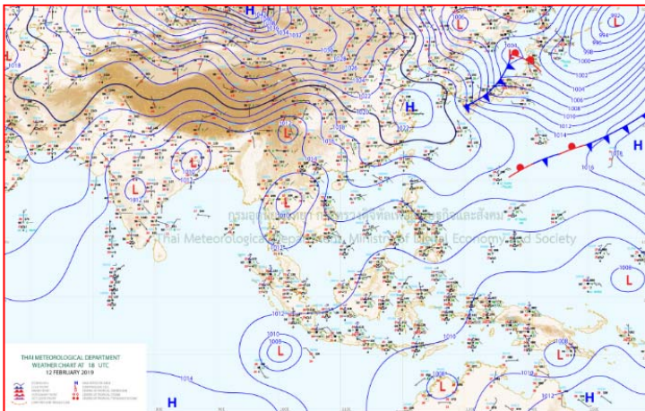
แผนที่อากาศ วันที่ ๑๓ มี.ค. ๒๕๖๒ เวลา ๐๑.๐๐ น.
