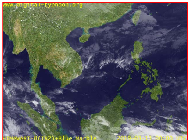
ภาพถ่ายดาวเทียม วันที่ ๑๓ มี.ค. ๒๕๖๒ เวลา ๐๗.๐๐ น.
