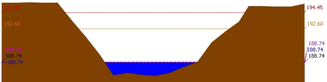
▲ ระดับปัจจุบัน --- ระดับวิกฤติ --- ระดับฝายระวัง ---- เมื่อวาน 7:00 น. - - - - - คาดการณ์ล่วงหน้า 1 วัน สถานี 120901T ห้วยมวกเหล็กที่ อ.มวกเหล็ก ต.มวกเหล็ก อ.มวกเหล็ก จ.สระบุรี ระดับน้ำ 188.74 ม.รทก.
