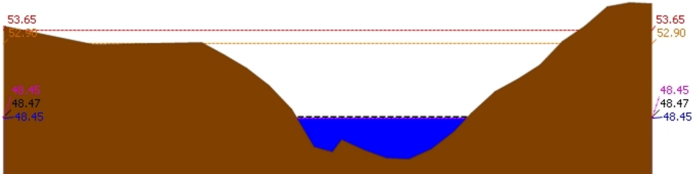
▲ ระดับปัจจุบัน --- ระดับวิกฤติ --- ระดับฝายระวัง ---- เมื่อวาน 7:00 น. - - - - - คาดการณ์ล่วงหน้า 1 วัน สถานี 120113T แม่น้ำป่าสักที่บ้านเขาค้าง ต.คลองกระจิง อ.ศรีเทพ จ.เพชรบูรณ์ ระดับน้ำ 48.45 ม.รทก.
