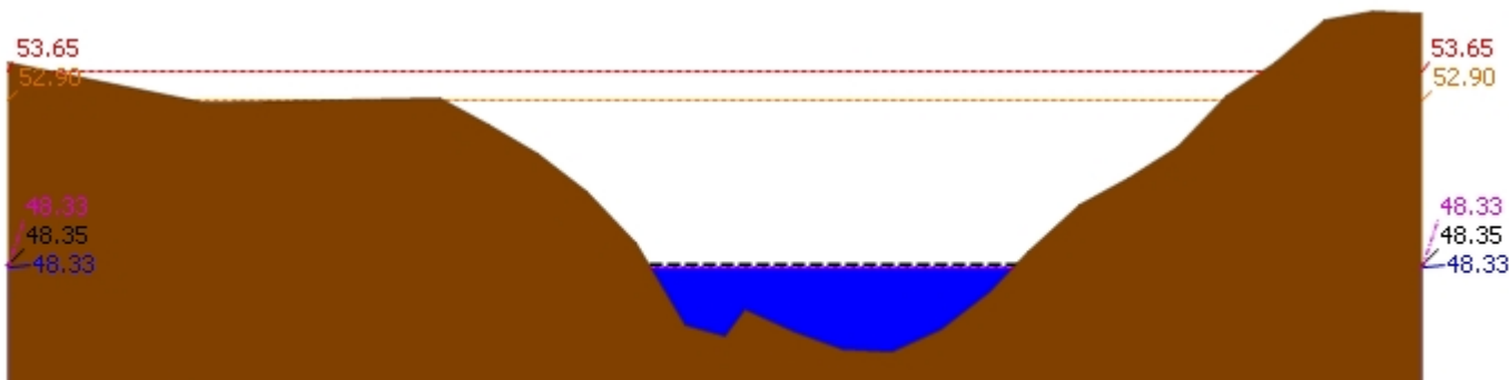
▲ ระดับปัจจุบัน --- ระดับวิกฤติ --- ระดับเฝ้าระวัง ---- เมื่อกาน 7:00 น. - - - - คาดการณ์ล่วงหน้า 1 วัน สถานี 120113T แม่น้ำป่าสักที่บ้านเขาค้าง ต.คลองกระจิง อ.ศรีเทพ จ.เพชรบูรณ์ ระดับน้ำ 48.33 ม.รทก.
