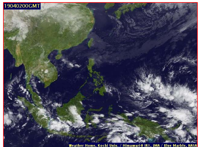
ภาพถ่ายดาวเทียม วันที่ ๒ เม.ย. ๒๕๖๒ เวลา ๐๗.๐๐ น.
