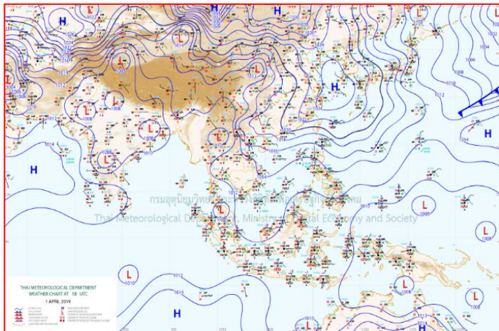
แผนที่อากาศ วันที่ ๒ เม.ย. ๒๕๖๒ เวลา ๐๖.๐๐ น.
