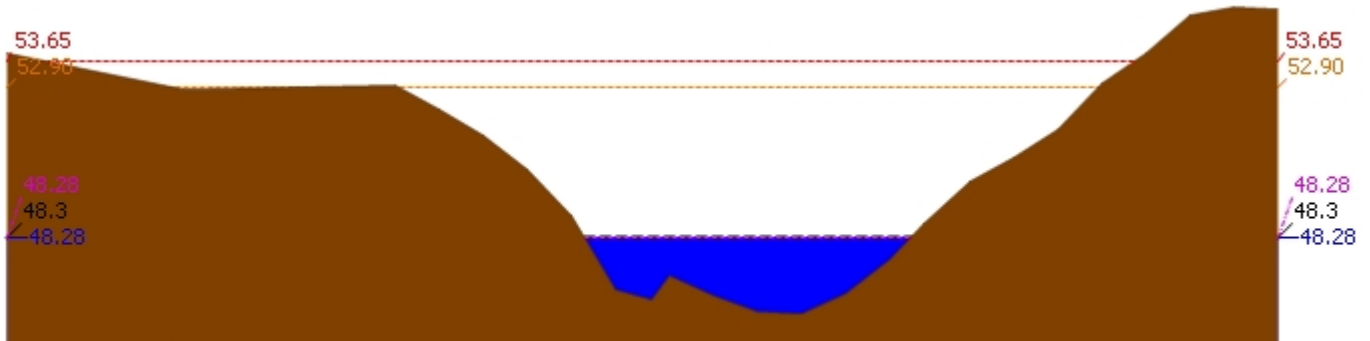
▲ ระดับปัจจุบัน --- ระดับวิกฤติ --- ระดับฝายระวัง ----- เมื่อวาน 7:00 น. - - - - - คาดการณ์ล่วงหน้า 1 วัน สถานี 120113T แม่น้ำป่าสักที่บ้านเขาค้าง ต.คลองกระจิง อ.ศรีเทพ จ.เพชรบูรณ์ ระดับน้ำ 48.28 ม.รทก.
