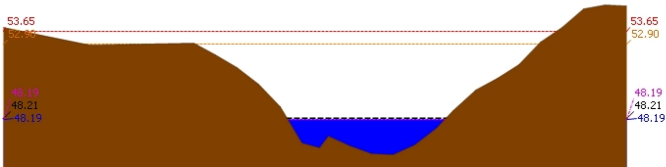
▲ ระดับปัจจุบัน --- ระดับวิกฤติ --- ระดับเขื่อน --- เมื่อวาน 7:00 น. --- คาดการณ์ล่วงหน้า 1 วัน สถานี 120113T แม่น้ำป่าสักที่บ้านเขาค้าง ต.คลองกระจิง อ.ศรีเทพ จ.เพชรบูรณ์ ระดับน้ำ 48.19 ม.รทก.
