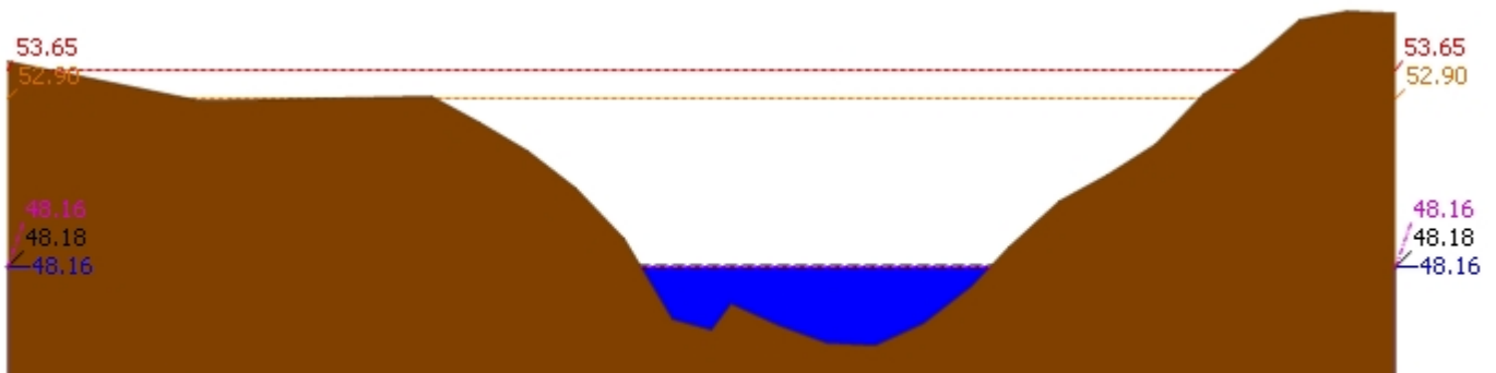
▲ ระดับปัจจุบัน --- ระดับวิกฤติ --- ระดับเฟิาระวัง ---- เมื่อกวาน 7:00 น. - - - - คาคการล้่างหน้า 1 วัน สถานี 120113T แม่น้ำป่าสักที่บ้านเขาค้าง ต.คลองกระจิง อ.ศรีเทพ จ.เพชรบูรณ์ ระดับน้ำ 48.16 ม.รทก.
