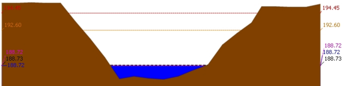
▲ ระดับปัจจุบัน --- ระดับวิกฤติ --- ระดับเฟิาระวัง ---- เมื่อกวาน 7:00 น. - - - - คาคการล้่างหน้า 1 วัน สถานี 120901T ทั่วมวกเหล็กที่ อ.มวกเหล็ก ต.มวกเหล็ก อ.มวกเหล็ก จ.สระบุรี ระดับน้ำ 188.72 ม.รทก.
