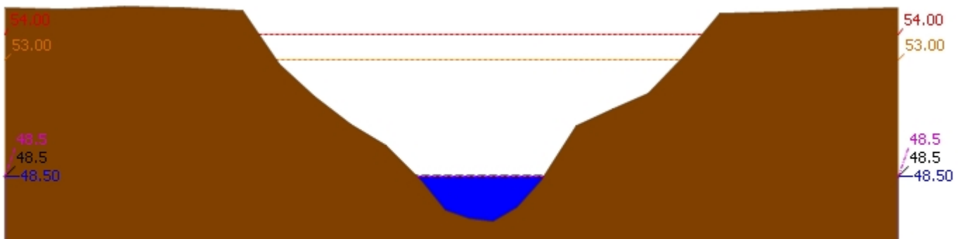
▲ ระดับปัจจุบัน --- ระดับวิกฤติ --- ระดับเฟิาระวัง ---- เมื่อกวาน 7:00 น. - - - - คาคการล้่างหน้า 1 วัน สถานี 120702T ลำสนธิที่บ้านท่ายาง ต.หนองขาหย่าง อ.ชัยบาดาล จ.ลพบุรี ระดับน้ำ 48.50 ม.รทก.
