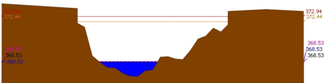
สถานี 060109T แม่น้ำปิงที่บ้านสบอ้อ ต.แม่บะ อ.เชียงดาว จ.เชียงใหม่ ระดับน้ำ 368.53 ม.รทก.
