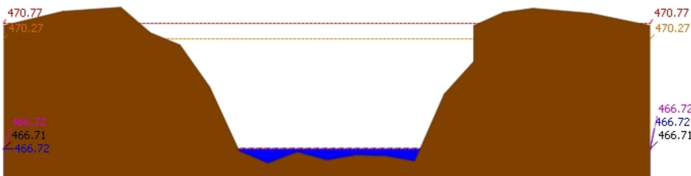
สถานี 061206T น้ำแม่แจ่มที่บ้านทัพ ต.ท่าผา อ.แม่แจ่ม จ.เชียงใหม่ ระดับน้ำ 466.72 ม.รทก.
