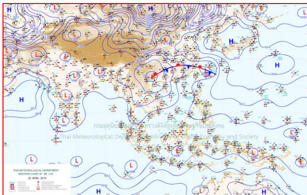
แผนที่อากาศ วันที่ 20 เม.ย. 2562 เวลา 07.00 น.
