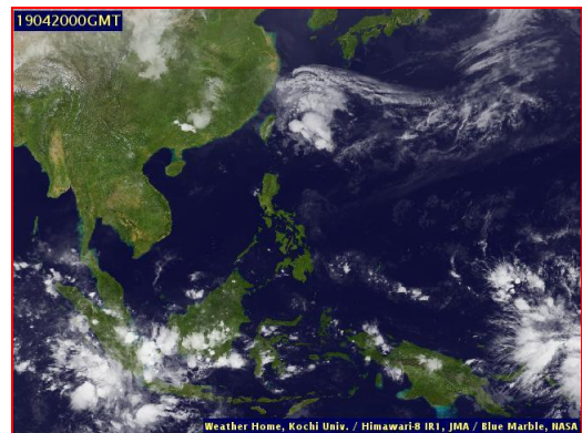
ภาพถ่ายจากดาวเทียม วันที่ 20 เม.ย. 2562
