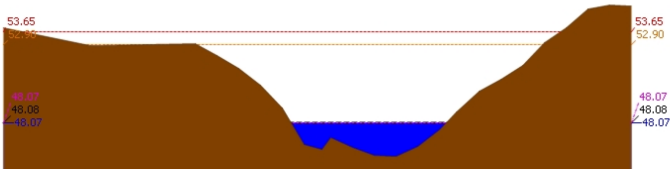
▲ ระดับปัจจุบัน --- ระดับวิกฤติ --- ระดับเฝ้าระวัง ---- เมื่อวาน 7:00 น. - - - - คาดการณ์ล่วงหน้า 1 วัน สถานี 120113T แม่น้ำป่าสักที่บ้านเขาค้าง ต.คลองกระจิง อ.ศรีเทพ จ.เพชรบูรณ์ ระดับน้ำ 48.07 ม.รทก.
