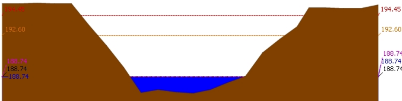
▲ ระดับปัจจุบัน --- ระดับวิกฤติ --- ระดับเฝ้าระวัง ---- เมื่อวาน 7:00 น. - - - - คาดการณ์ล่วงหน้า 1 วัน สถานี 120901T ห้วยมวกเหล็กที่ อ.มวกเหล็ก ต.มวกเหล็ก อ.มวกเหล็ก จ.สระบุรี ระดับน้ำ 188.74 ม.รทก.
