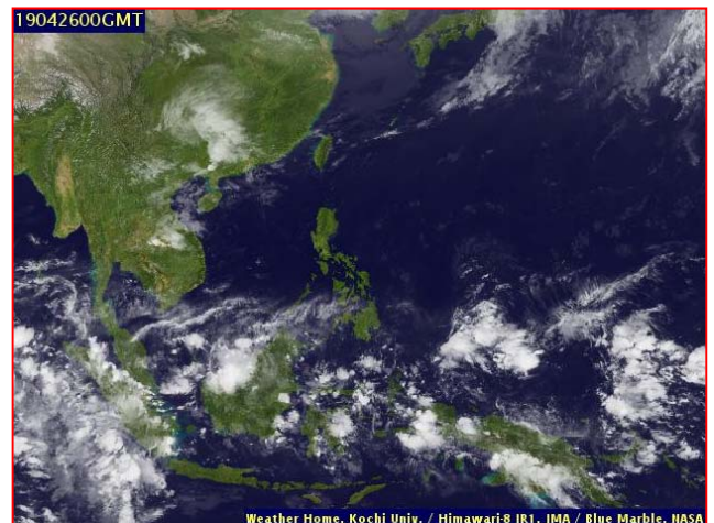
ภาพถ่ายดาวเทียม วันที่ ๒๖ เม.ย. ๒๕๖๒ เวลา ๐๗.๐๐ น.
