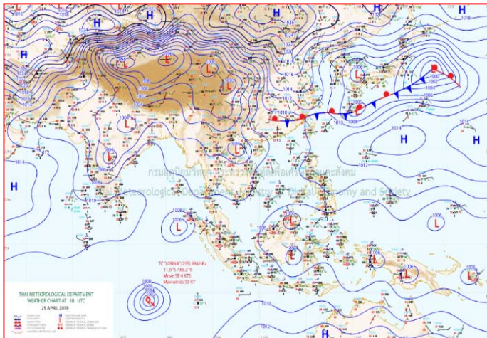
แผนที่อากาศ วันที่ ๒๖ เม.ย. ๒๕๖๒ เวลา ๐๖.๐๐ น.
